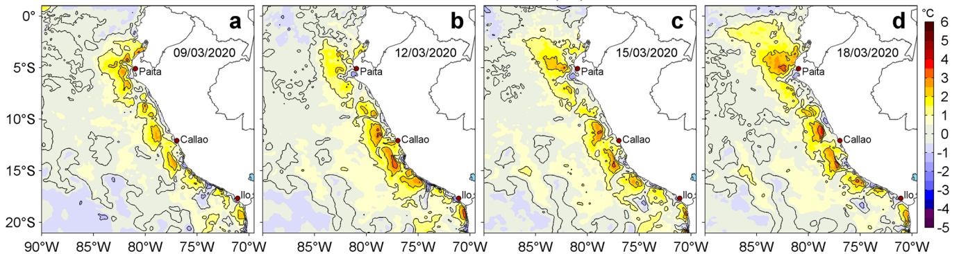
Figura 3. Anomalías de la temperatura superficial del mar (TSM, °C) para los días: a) 09, b) 12, c) 15 y d) 18 de marzo de 2020. Las anomalías se calcularon respecto de la climatología para el periodo 2007-2016. Datos: OSTIA-UKMO-L4-GLOB-v2.0 (UK Met Office, 2012; Donlon et al, 2012). Procesamiento: LHF/AFIOF/DGIOCC/IMARPE.
