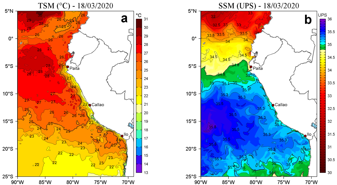
Figura 2. a) Temperatura superficial del mar (TSM, °C) y b) Salinidad superficial del mar (SSM, UPS), para el 18 de marzo de 2020. Datos: OSTIA-UKMO-L4-GLOB-v2.0 (UK Met Office, 2012; Donlon et al, 2012) disponible en https://podaac.jpl.nasa.gov/dataset/OSTIA-UKMO-L4-GLOB-v2.0 para (a) y Hybrid Coordinate Ocean Model v. GOFS 3.1 (HYCOM; Halliwell et al., 1998; 2000; Bleck, 2001) para (b). Procesamiento: LHF/AFIOF/DGIOCC/IMARPE.
