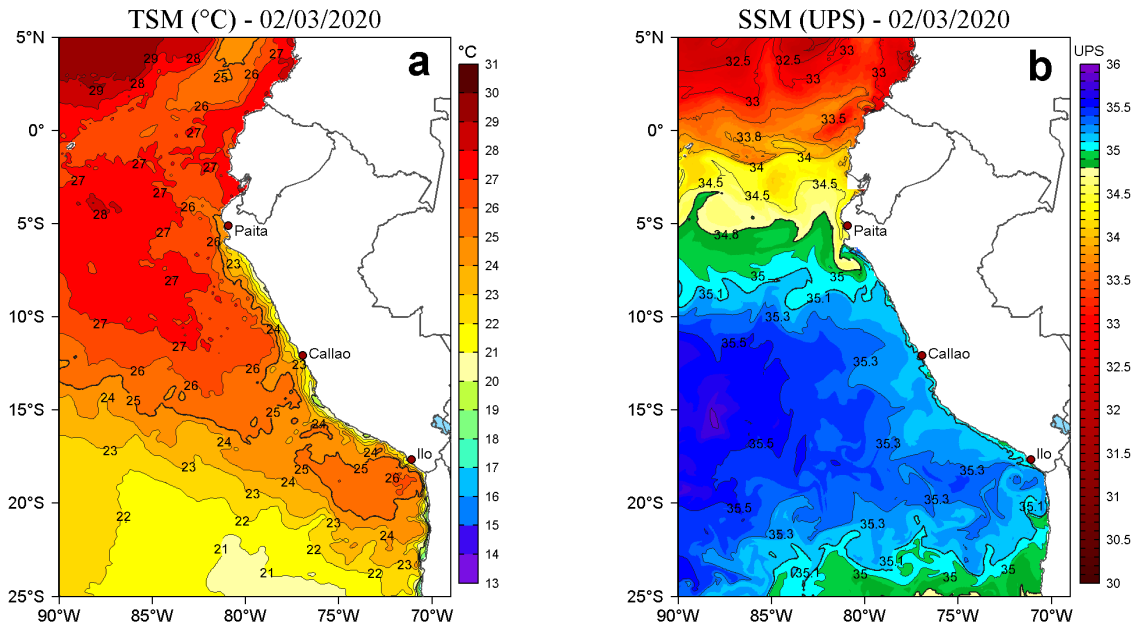
Figura 2. a) Temperatura superficial del mar (TSM, °C) y b) Salinidad superficial del mar (SSM, UPS), para el 02 de marzo de 2020. Datos: OSTIA-UKMO-L4-GLOB-v2.0 (UK Met Office, 2012; Donlon et al, 2012) disponible en https://podaac.jpl.nasa.gov/dataset/OSTIA-UKMO-L4-GLOB-v2.0 para (a) y Hybrid Coordinate Ocean Model v. GOF5 3.1 (HYCOM; Halliwell et al., 1998; 2000; Bleck, 2001) para (b). Procesamiento: LHF/AFIOF/DGIOCC/IMARPE.
