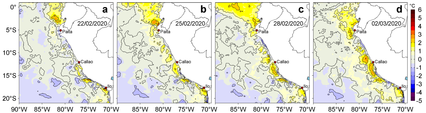
Figura 3. Anomalías de la temperatura superficial del mar (TSM, °C) para los días: a) 22, b) 25 y c) 28 de febrero y d) 02 de marzo de 2020. Las anomalías se calcularon respecto de la climatología para el periodo 2007-2016. Datos: OSTIA-UKMO-L4-GLOB-v2.0 (UK Met Office, 2012; Donlon et al, 2012). Procesamiento: LHF/AFIOF/DGIOCC/IMARPE.
