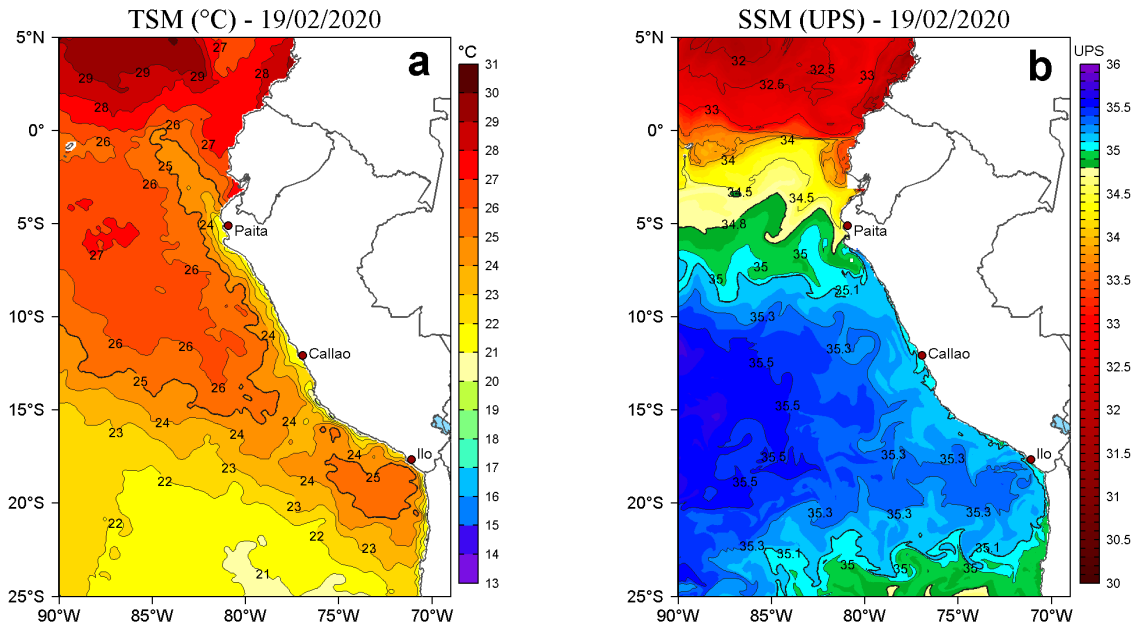
Figura 2. a) Temperatura superficial del mar (TSM, °C) y b) Salinidad superficial del mar (SSM, UPS), para el 19 de febrero de 2020. Datos: OSTIA-UKMO-L4-GLOB-v2.0 (UK Met Office, 2012; Donlon et al, 2012) disponible en https://podaac.jpl.nasa.gov/dataset/OSTIA-UKMO-L4-GLOB-v2.0 para (a) y Hybrid Coordinate Ocean Model v. GOF3 3.1 (HYCOM; Halliwell et al., 1998; 2000; Bleck, 2001) para (b). Procesamiento: LHF/AFIOF/DGIOCC/IMARPE.
