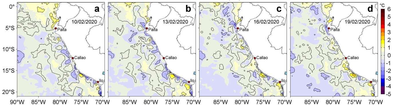
Figura 3. Anomalías de la temperatura superficial del mar (TSM, °C) para los días: a) 10, b) 13, c) 16 y d) 19 de febrero de 2020. Las anomalías se calcularon respecto de la climatología para el periodo 2007-2016. Datos: OSTIA-UKMO-L4-GLOB-v2.0 (UK Met Office, 2012; Donlon et al, 2012). Procesamiento: LHF/AFIOF/DGIOCC/IMARPE.
