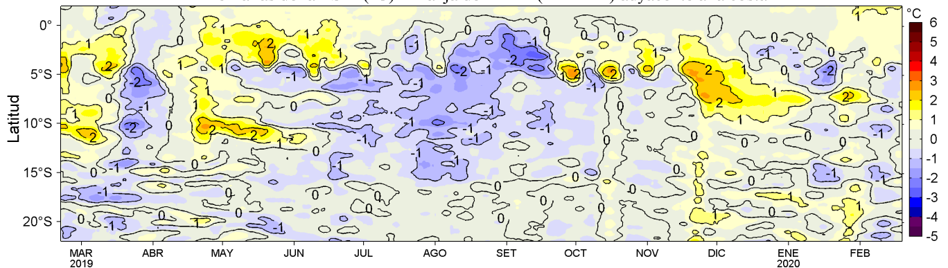
Figura 4. Variación promedio de las anomalías de la temperatura superficial del mar (TSM, °C) para una franja de 60 mn (~111 km) adyacente al litoral peruano para los últimos doce meses al 19 de febrero de 2020. Datos: OSTIA-UKMO-L4-GLOB-v2.0 (UK Met. Office, 2012; Donlon et al, 2012) disponible en https://podaac.jpl.nasa.gov/dataset/OSTIA-UKMO-L4-GLOB-v2.0 . Las anomalías se calcularon con respecto al periodo 2007-2016. Procesamiento: LHF/AFIOF/DGIOCC/IMARPE.
