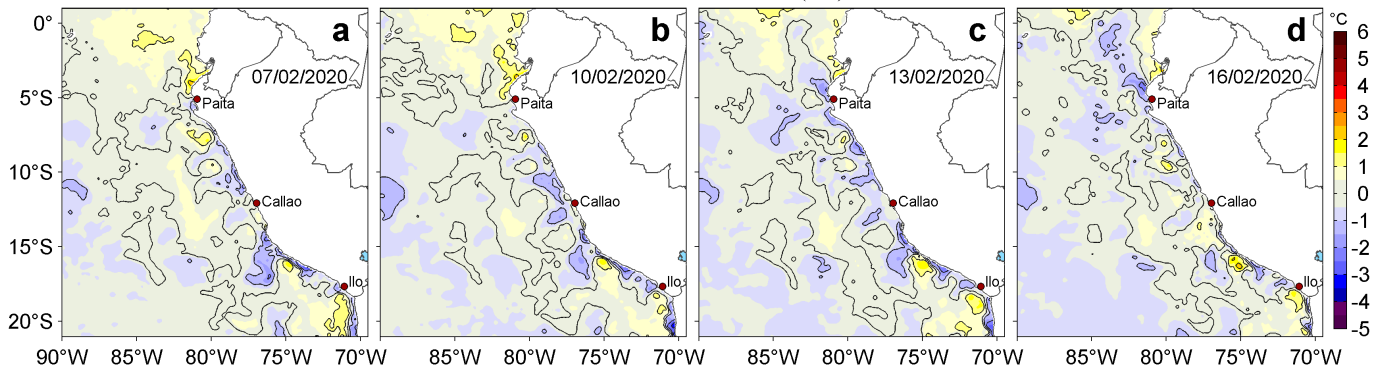
Figura 3. Anomalías de la temperatura superficial del mar (TSM, °C) para los días: a) 07, b) 10, c) 13 y d) 16 de febrero de 2020. Las anomalías se calcularon respecto de la climatología para el periodo 2007-2016. Datos: OSTIA-UKMO-L4-GLOB-v2.0 (UK Met Office, 2012; Donlon et al, 2012). Procesamiento: LHF/AFIOF/DGIOCC/IMARPE.
