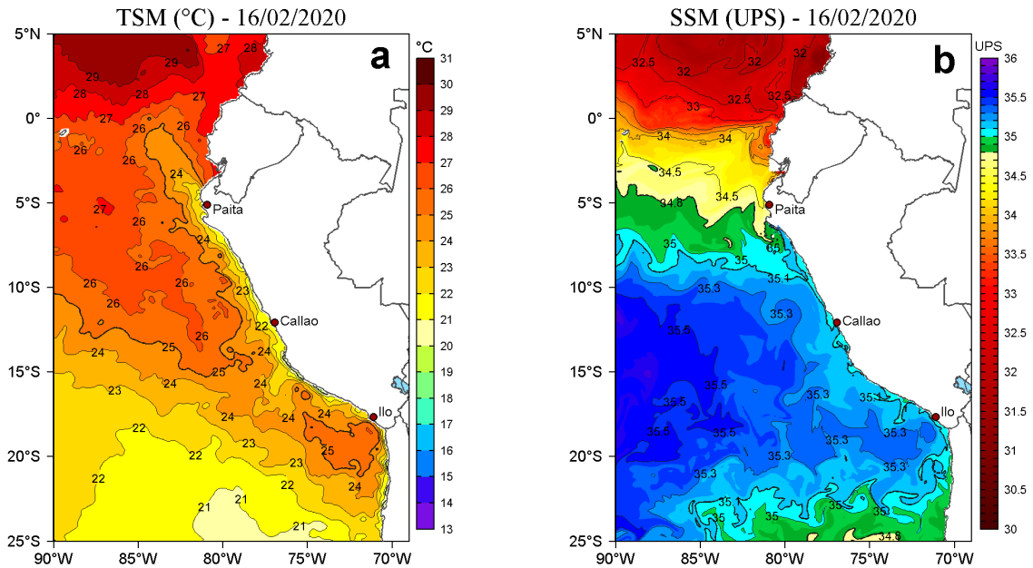
Figura 2. a) Temperatura superficial del mar (TSM, °C) y b) Salinidad superficial del mar (SSM, UPS), para el 16 de febrero de 2020. Datos: OSTIA-UKMO-L4-GLOB-v2.0 (UK Met Office, 2012; Donlon et al, 2012) disponible en https://podaac.jpl.nasa.gov/dataset/OSTIA-UKMO-L4-GLOB-v2.0 para (a) y Hybrid Coordinate Ocean Model v. GOF3 3.1 (HYCOM; Halliwell et al., 1998; 2000; Bleck, 2001) para (b). Procesamiento: LHF/AFIOF/DGIOCC/IMARPE.
