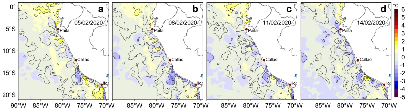
Figura 3. Anomalías de la temperatura superficial del mar (TSM, °C) para los días: a) 05, b) 08, c) 11 y d) 14 de febrero de 2020. Las anomalías se calcularon respecto de la climatología para el periodo 2007-2016. Datos: OSTIA-UKMO-L4-GLOB-v2.0 (UK Met Office, 2012; Donlon et al, 2012). Procesamiento: LHF/AFIOF/DGIOCC/IMARPE.
