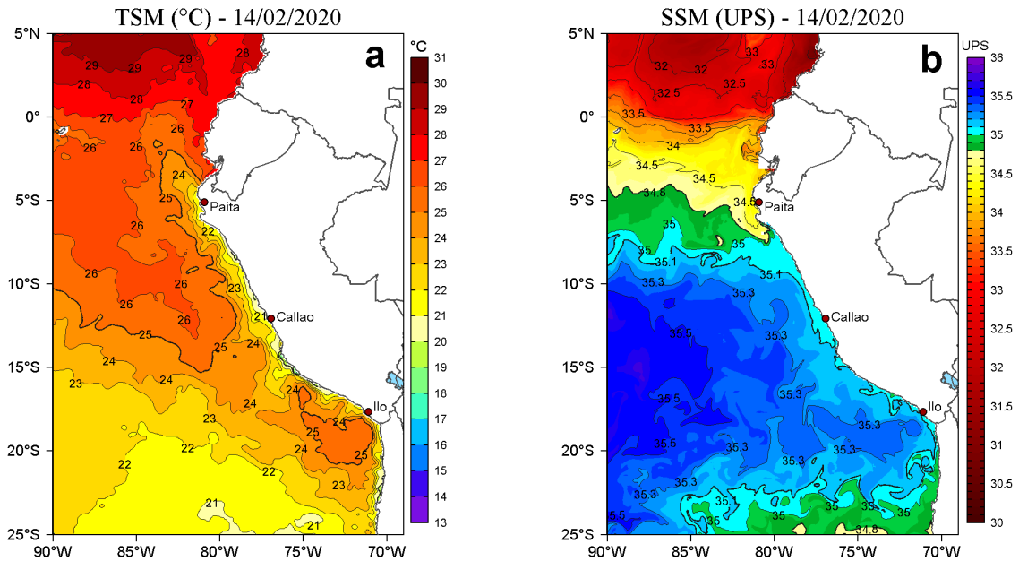
Figura 2. a) Temperatura superficial del mar (TSM, °C) y b) Salinidad superficial del mar (SSM, UPS), para el 14 de febrero de 2020. Datos: OSTIA-UKMO-L4-GLOB-v2.0 (UK Met Office, 2012; Donlon et al, 2012) disponible en https://podaac.jpl.nasa.gov/dataset/OSTIA-UKMO-L4-GLOB-v2.0 para (a) y Hybrid Coordinate Ocean Model v. GOF3 3.1 (HYCOM; Halliwell et al., 1998; 2000; Bleck, 2001) para (b). Procesamiento: LHF/AFIOF/DGIOCC/IMARPE.
