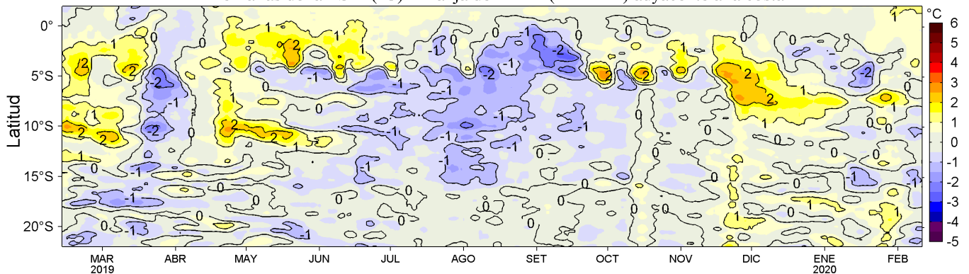
Figura 4. Variación promedio de las anomalías de la temperatura superficial del mar (TSM, °C) para una franja de 60 mn (~111 km) adyacente al litoral peruano para los últimos doce meses al 11 de febrero de 2020. Datos: OSTIA-UKMO-L4-GLOB-v2.0 (UK Met. Office, 2012; Donlon et al, 2012) disponible en https://podaac.jpl.nasa.gov/dataset/OSTIA-UKMO-L4-GLOB-v2.0 . Las anomalías se calcularon con respecto al periodo 2007-2016. Procesamiento: LHF/AFIOF/DGIOCC/IMARPE.
