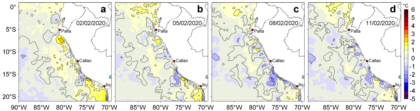
Figura 3. Anomalías de la temperatura superficial del mar (TSM, °C) para los días: a) 02, b) 05, c) 08 y d) 11 de febrero de 2020. Las anomalías se calcularon respecto de la climatología para el periodo 2007-2016. Datos: OSTIA-UKMO-L4-GLOB-v2.0 (UK Met Office, 2012; Donlon et al, 2012). Procesamiento: LHF/AFIOF/DGIOCC/IMARPE.
