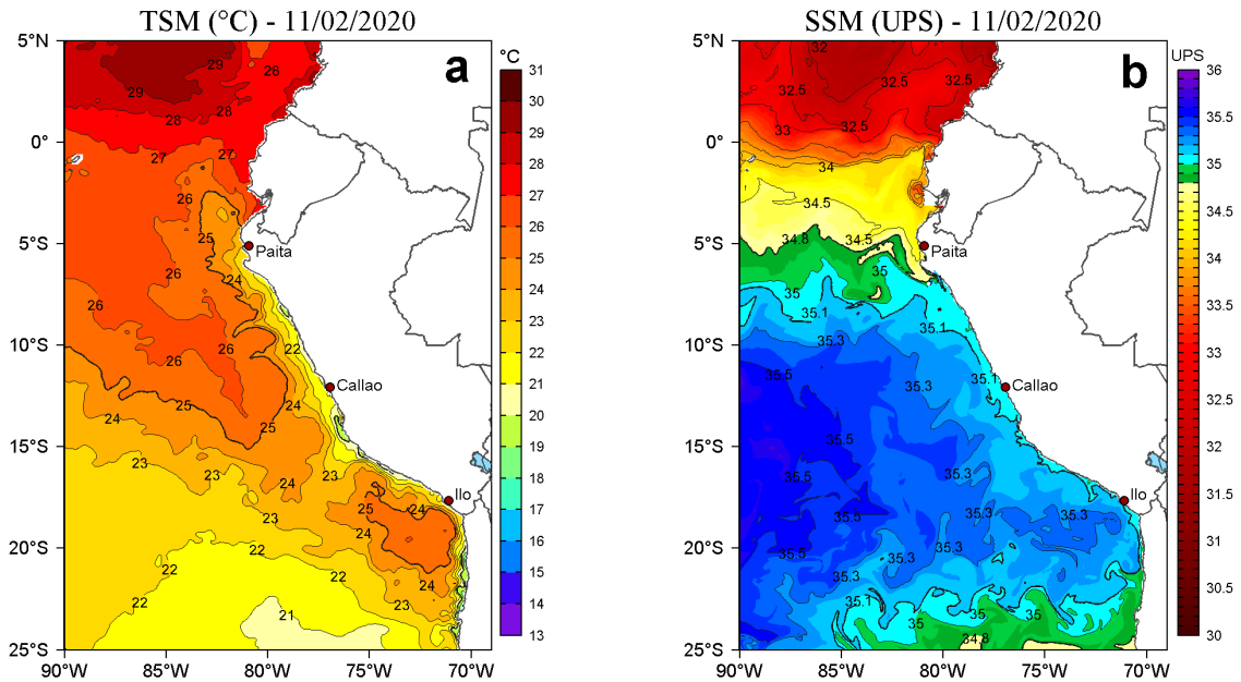
Figura 2. a) Temperatura superficial del mar (TSM, °C) y b) Salinidad superficial del mar (SSM, UPS), para el 11 de febrero de 2020. Datos: OSTIA-UKMO-L4-GLOB-v2.0 (UK Met Office, 2012; Donlon et al, 2012) disponible en https://podaac.jpl.nasa.gov/dataset/OSTIA-UKMO-L4-GLOB-v2.0 para (a) y Hybrid Coordinate Ocean Model v. GOF3 3.1 (HYCOM; Halliwell et al., 1998; 2000; Bleck, 2001) para (b). Procesamiento: LHF/AFIOF/DGIOCC/IMARPE.
