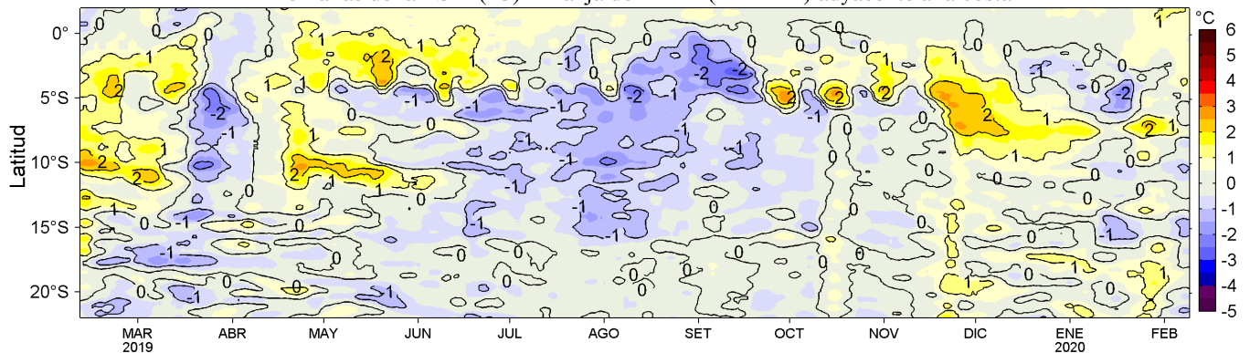
Figura 4. Variación promedio de las anomalías de la temperatura superficial del mar (TSM, °C) para una franja de 60 mn (~111 km) adyacente al litoral peruano para los últimos doce meses al 09 de febrero de 2020. Datos: OSTIA-UKMO-L4-GLOB-v2.0 (UK Met. Office, 2012; Donlon et al, 2012) disponible en https://podaac.jpl.nasa.gov/dataset/OSTIA-UKMO-L4-GLOB-v2.0 . Las anomalías se calcularon con respecto al periodo 2007-2016. Procesamiento: LHF/AFIOF/DGIOCC/IMARPE.
