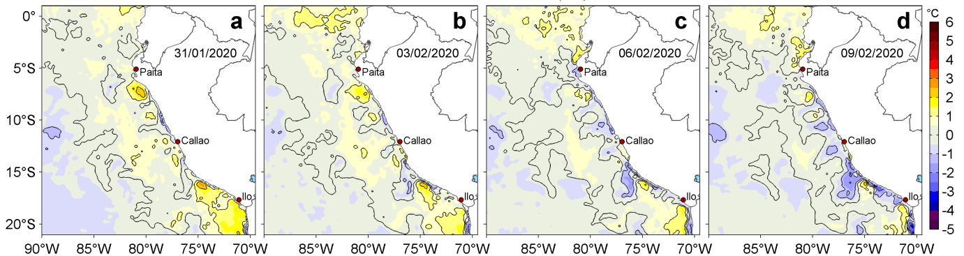
Figura 3. Anomalías de la temperatura superficial del mar (TSM, °C) para los días: a) 31 de enero, b) 03, c) 06 y d) 09 de febrero de 2020. Las anomalías se calcularon respecto de la climatología para el periodo 2007-2016. Datos: OSTIA-UKMO-L4-GLOB-v2.0 (UK Met Office, 2012; Donlon et al, 2012). Procesamiento: LHF/AFIOF/DGIOCC/IMARPE.
