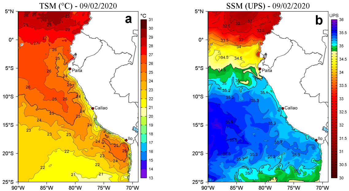
Figura 2. a) Temperatura superficial del mar (TSM, °C) y b) Salinidad superficial del mar (SSM, UPS), para el 09 de febrero de 2020. Datos: OSTIA-UKMO-L4-GLOB-v2.0 (UK Met Office, 2012; Donlon et al, 2012) disponible en https://podaac.jpl.nasa.gov/dataset/OSTIA-UKMO-L4-GLOB-v2.0 para (a) y Hybrid Coordinate Ocean Model v. GOF3 3.1 (HYCOM; Halliwell et al., 1998; 2000; Bleck, 2001) para (b). Procesamiento: LHF/AFIOF/DGIOCC/IMARPE.
