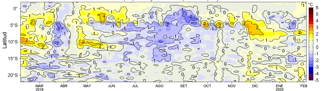
Figura 4. Variación promedio de las anomalías de la temperatura superficial del mar (TSM, °C) para una franja de 60 mn (~111 km) adyacente al litoral peruano para los últimos doce meses al 04 de febrero de 2020. Datos: OSTIA-UKMO-L4-GLOB-v2.0 (UK Met. Office, 2012; Donlon et al, 2012) disponible en https://podaac.jpl.nasa.gov/dataset/OSTIA-UKMO-L4-GLOB-v2.0 . Las anomalías se calcularon con respecto al periodo 2007-2016. Procesamiento: LHF/AFIOF/DGIOCC/IMARPE.
