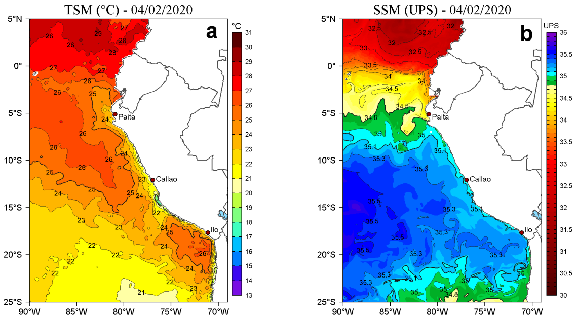
Figura 2. a) Temperatura superficial del mar (TSM, °C) y b) Salinidad superficial del mar (SSM, UPS), para el 04 de febrero de 2020. Datos: OSTIA-UKMO-L4-GLOB-v2.0 (UK Met Office, 2012; Donlon et al, 2012) disponible en https://podaac.jpl.nasa.gov/dataset/OSTIA-UKMO-L4-GLOB-v2.0 para (a) y Hybrid Coordinate Ocean Model v. GOF3 3.1 (HYCOM; Halliwell et al., 1998; 2000; Bleck, 2001) para (b). Procesamiento: LHF/AFIOF/DGIOCC/IMARPE.
