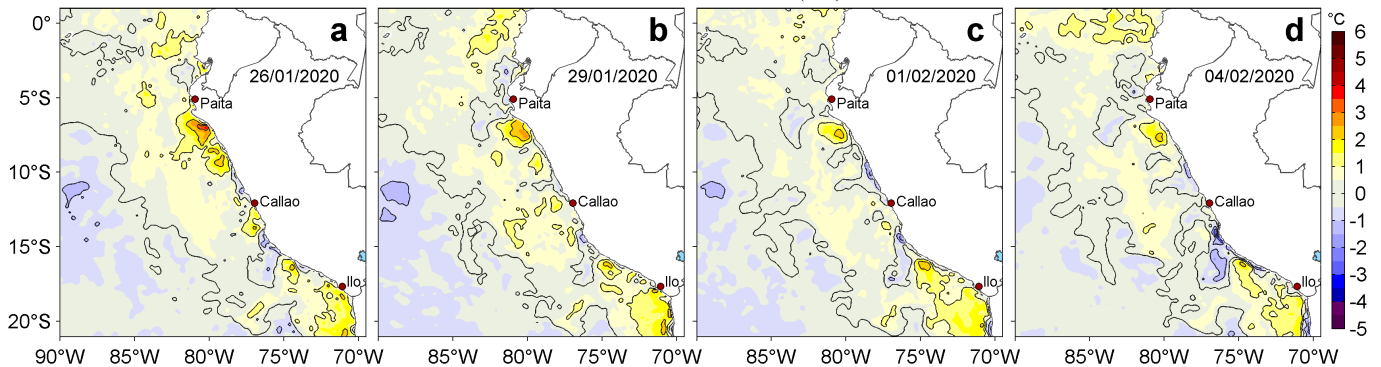
Figura 3. Anomalías de la temperatura superficial del mar (TSM, °C) para los días: a) 26 y b) 29 de enero, c) 01 y d) 04 de febrero de 2020. Las anomalías se calcularon respecto de la climatología para el periodo 2007-2016. Datos: OSTIA-UKMO-L4-GLOB-v2.0 (UK Met Office, 2012; Donlon et al, 2012). Procesamiento: LHF/AFIOF/DGIOCC/IMARPE.
