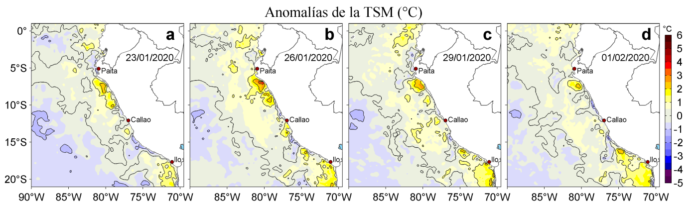
Figura 3. Anomalías de la temperatura superficial del mar (TSM, °C) para los días: a) 23, b) 26 y c) 29 de enero y d) 01 de febrero de 2020. Las anomalías se calcularon respecto de la climatología para el periodo 2007-2016. Datos: OSTIA-UKMO-L4-GLOB-v2.0 (UK Met Office, 2012; Donlon et al, 2012). Procesamiento: LHF/AFIOF/DGIOCC/IMARPE.
