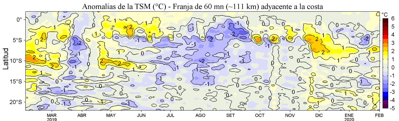
Figura 4. Variación promedio de las anomalías de la temperatura superficial del mar (TSM, °C) para una franja de 60 mn (~111 km) adyacente al litoral peruano para los últimos doce meses al 01 de febrero de 2020. Datos: OSTIA-UKMO-L4-GLOB-v2.0 (UK Met. Office, 2012; Donlon et al, 2012) disponible en https://podaac.jpl.nasa.gov/dataset/OSTIA-UKMO-L4-GLOB-v2.0 . Las anomalías se calcularon con respecto al periodo 2007-2016. Procesamiento: LHF/AFIOF/DGIOCC/IMARPE.
