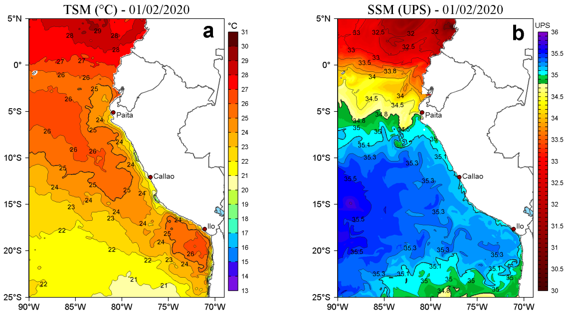
Figura 2. a) Temperatura superficial del mar (TSM, °C) y b) Salinidad superficial del mar (SSM, UPS), para el 01 de febrero de 2020. Datos: OSTIA-UKMO-L4-GLOB-v2.0 (UK Met Office, 2012; Donlon et al, 2012) disponible en https://podaac.jpl.nasa.gov/dataset/OSTIA-UKMO-L4-GLOB-v2.0 para (a) y Hybrid Coordinate Ocean Model v. GOF3 3.1 (HYCOM; Halliwell et al., 1998; 2000; Bleck, 2001) para (b). Procesamiento: LHF/AFIOF/DGIOCC/IMARPE.
