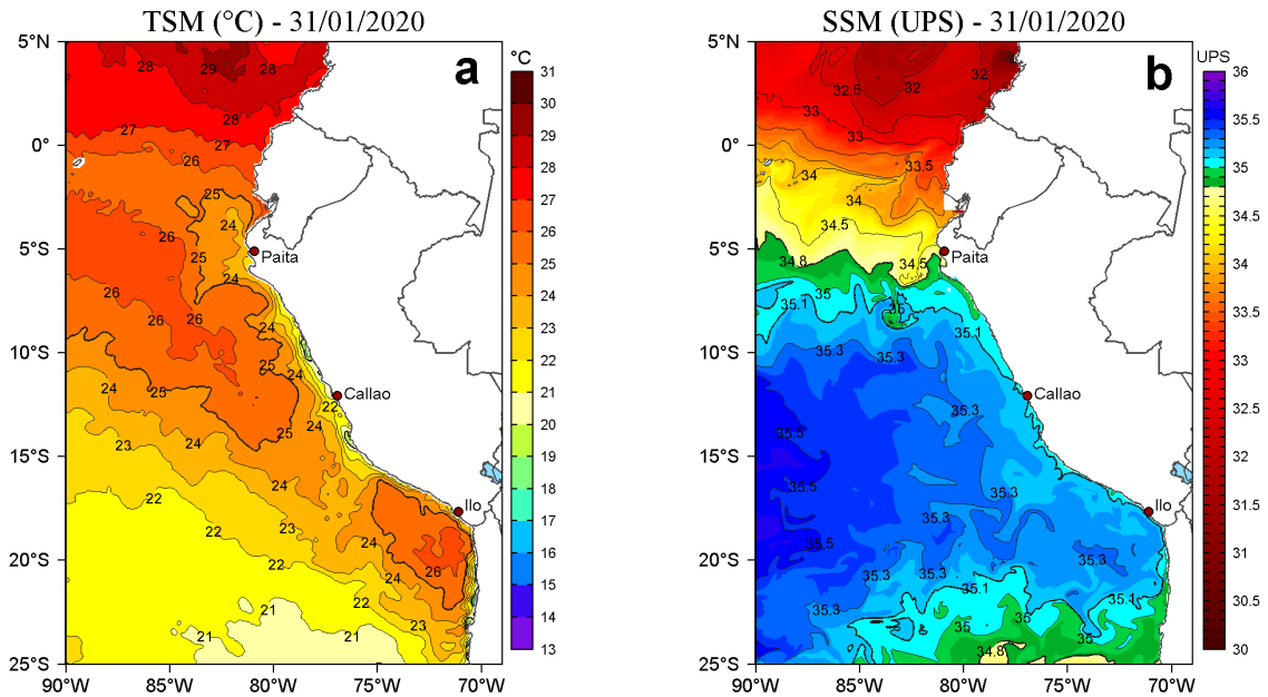
Figura 2. a) Temperatura superficial del mar (TSM, °C) y b) Salinidad superficial del mar (SSM, UPS), para el 31 de enero de 2020. Datos: OSTIA-UKMO-L4-GLOB-v2.0 (UK Met Office, 2012; Donlon et al, 2012) disponible en https://podaac.jpl.nasa.gov/dataset/OSTIA-UKMO-L4-GLOB-v2.0 para (a) y Hybrid Coordinate Ocean Model v. GOF5 3.1 (HYCOM; Halliwell et al., 1998; 2000; Bleck, 2001) para (b). Procesamiento: LHF/AFIOF/DGIOCC/IMARPE.
