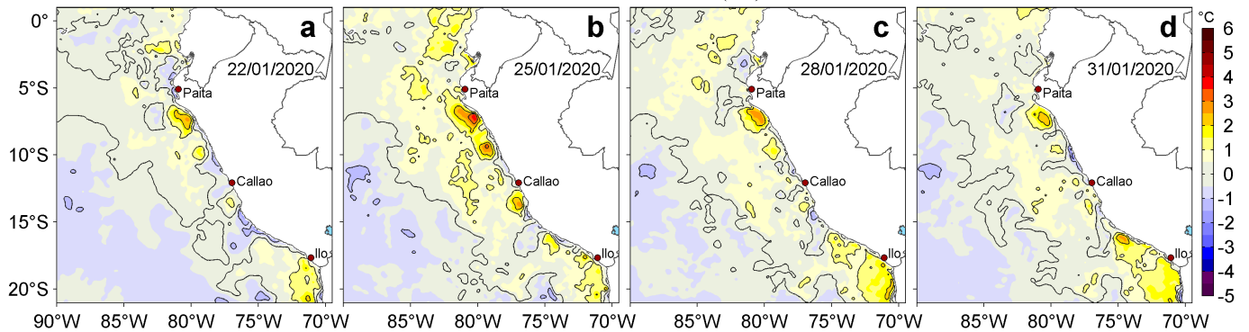
Figura 3. Anomalías de la temperatura superficial del mar (TSM, °C) para los días: a) 22, b) 25, c) 28 y d) 31 de enero de 2020. Las anomalías se calcularon respecto de la climatología para el periodo 2007-2016. Datos: OSTIA-UKMO-L4-GLOB-v2.0 (UK Met Office, 2012; Donlon et al, 2012). Procesamiento: LHF/AFIOF/DGIOCC/IMARPE.
