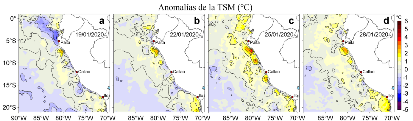
Figura 3. Anomalías de la temperatura superficial del mar (TSM, °C) para los días: a) 19, b) 22, c) 25 y d) 28 de enero de 2020. Las anomalías se calcularon respecto de la climatología para el periodo 2007-2016. Datos: OSTIA-UKMO-L4-GLOB-v2.0 (UK Met Office, 2012; Donlon et al, 2012). Procesamiento: LHFH/AFIOF/DGIOCC/IMARPE.
