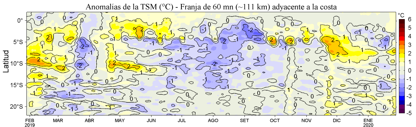
Figura 4. Variación promedio de las anomalías de la temperatura superficial del mar (TSM, °C) para una franja de 60 mn (~111 km) adyacente al litoral peruano para los últimos doce meses al 28 de enero de 2020. Datos: OSTIA-UKMO-L4-GLOB-v2.0 (UK Met. Office, 2012; Donlon et al, 2012) disponible en https://podaac.jpl.nasa.gov/dataset/OSTIA-UKMO-L4-GLOB-v2.0 . Las anomalías se calcularon con respecto al periodo 2007-2016. Procesamiento: LHFH/AFIOF/DGIOCC/IMARPE.
