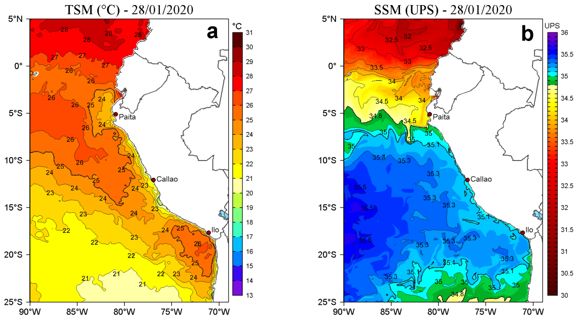
Figura 2. a) Temperatura superficial del mar (TSM, °C) y b) Salinidad superficial del mar (SSM, UPS), para el 28 de enero de 2020. Datos: OSTIA-UKMO-L4-GLOB-v2.0 (UK Met Office, 2012; Donlon et al, 2012) disponible en https://podaac.jpl.nasa.gov/dataset/OSTIA-UKMO-L4-GLOB-v2.0 para (a) y Hybrid Coordinate Ocean Model v. GOFS 3.1 (HYCOM; Halliwell et al., 1998; 2000; Bleck, 2001) para (b). Procesamiento: LHFH/AFIOF/DGIOCC/IMARPE.
