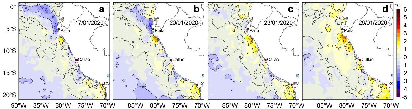
Figura 3. Anomalías de la temperatura superficial del mar (TSM, °C) para los días: a) 17, b) 20, c) 23 y d) 26 de enero de 2020. Las anomalías se calcularon respecto de la climatología para el periodo 2007-2016. Datos: OSTIA-UKMO-L4-GLOB-v2.0 (UK Met Office, 2012; Donlon et al, 2012). Procesamiento: LHF/AFIOF/DGIOCC/IMARPE.
