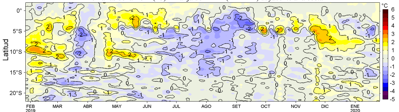
Figura 4. Variación promedio de las anomalías de la temperatura superficial del mar (TSM, °C) para una franja de 60 mn (~111 km) adyacente al litoral peruano para los últimos doce meses al 26 de enero de 2020. Datos: OSTIA-UKMO-L4-GLOB-v2.0 (UK Met. Office, 2012; Donlon et al, 2012) disponible en https://podaac.jpl.nasa.gov/dataset/OSTIA-UKMO-L4-GLOB-v2.0 . Las anomalías se calcularon con respecto al periodo 2007-2016. Procesamiento: LHF/AFIOF/DGIOCC/IMARPE.
