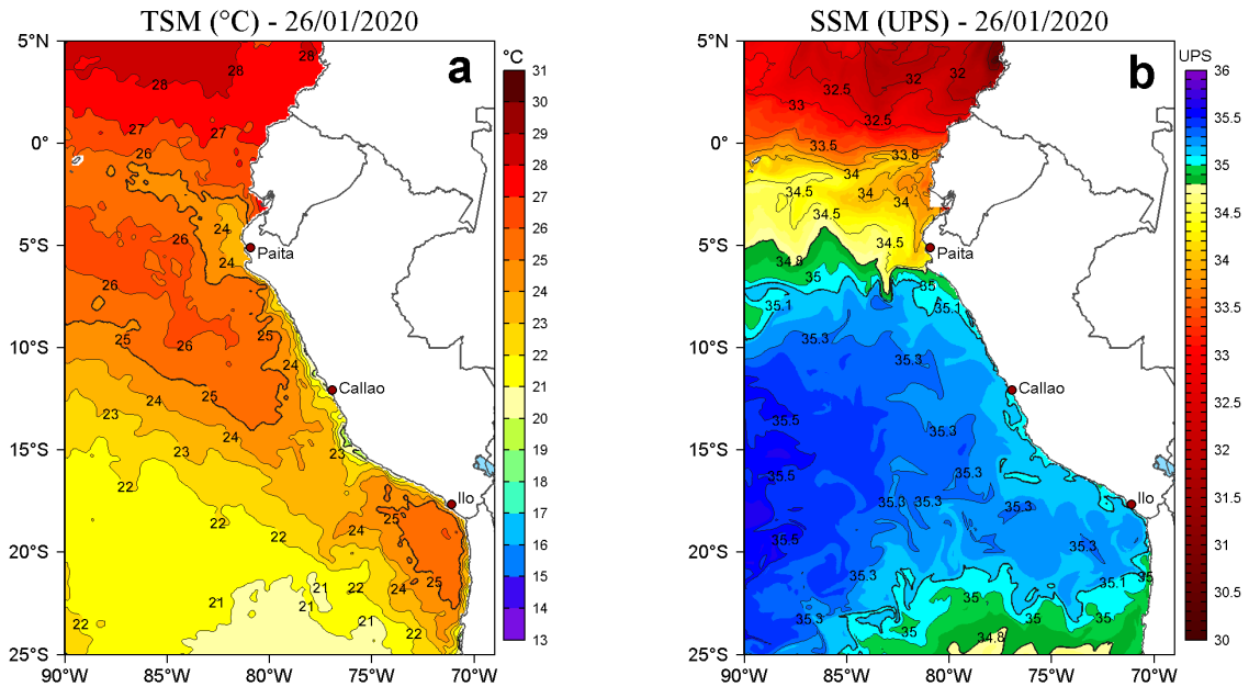
Figura 2. a) Temperatura superficial del mar (TSM, °C) y b) Salinidad superficial del mar (SSM, UPS), para el 26 de enero de 2020. Datos: OSTIA-UKMO-L4-GLOB-v2.0 (UK Met Office, 2012; Donlon et al, 2012) disponible en https://podaac.jpl.nasa.gov/dataset/OSTIA-UKMO-L4-GLOB-v2.0 para (a) y Hybrid Coordinate Ocean Model v. GOF3 3.1 (HYCOM; Halliwell et al., 1998; 2000; Bleck, 2001) para (b). Procesamiento: LHF/AFIOF/DGIOCC/IMARPE.
