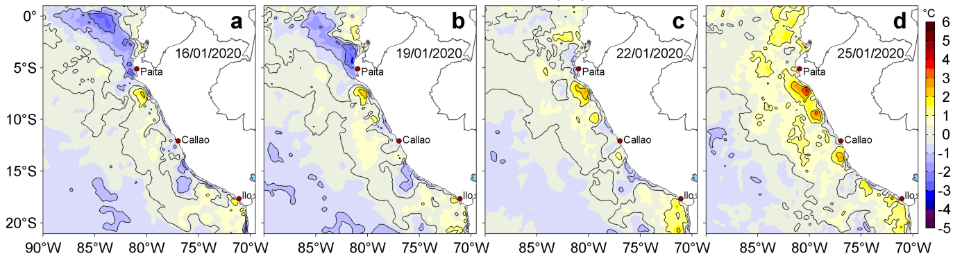
Figura 3. Anomalías de la temperatura superficial del mar (TSM, °C) para los días: a) 16, b) 19, c) 22 y d) 25 de enero de 2020. Las anomalías se calcularon respecto de la climatología para el periodo 2007-2016. Datos: OSTIA-UKMO-L4-GLOB-v2.0 (UK Met Office, 2012; Donlon et al, 2012). Procesamiento: LHFM/AFIOF/DGIOCC/IMARPE.
