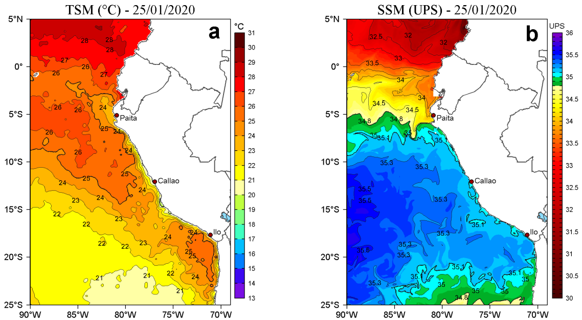
Figura 2. a) Temperatura superficial del mar (TSM, °C) y b) Salinidad superficial del mar (SSM, UPS), para el 25 de enero de 2020. Datos: OSTIA-UKMO-L4-GLOB-v2.0 (UK Met Office, 2012; Donlon et al, 2012) disponible en https://podaac.jpl.nasa.gov/dataset/OSTIA-UKMO-L4-GLOB-v2.0 para (a) y Hybrid Coordinate Ocean Model v. GOF3 3.1 (HYCOM; Halliwell et al., 1998; 2000; Bleck, 2001) para (b). Procesamiento: LHFM/AFIOF/DGIOCC/IMARPE.
