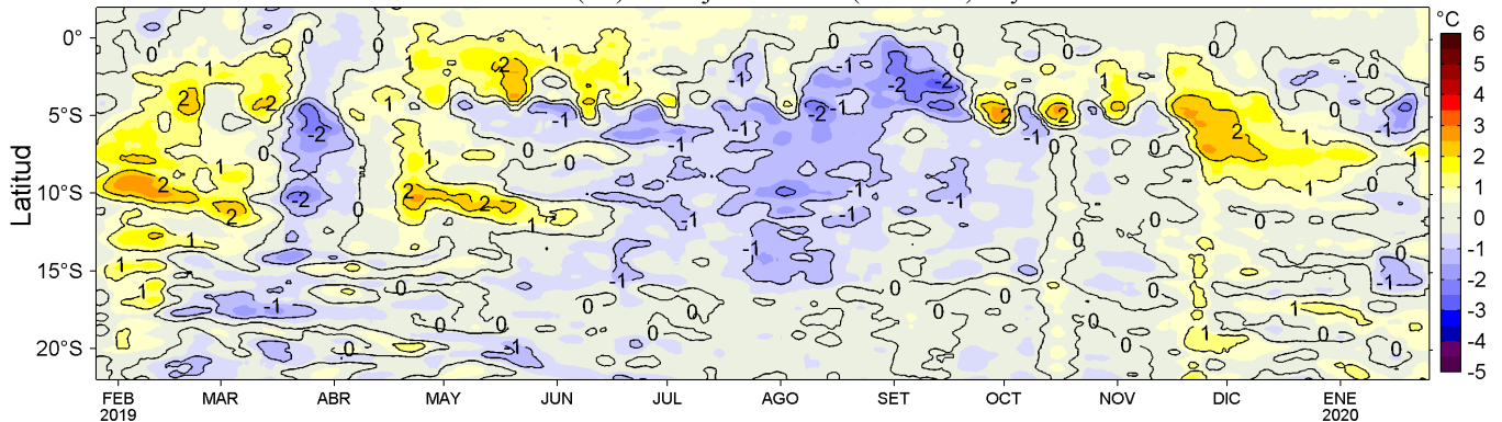
Figura 4. Variación promedio de las anomalías de la temperatura superficial del mar (TSM, °C) para una franja de 60 mn (~111 km) adyacente al litoral peruano para los últimos doce meses al 25 de enero de 2020. Datos: OSTIA-UKMO-L4-GLOB-v2.0 (UK Met. Office, 2012; Donlon et al, 2012) disponible en https://podaac.jpl.nasa.gov/dataset/OSTIA-UKMO-L4-GLOB-v2.0 . Las anomalías se calcularon con respecto al periodo 2007-2016. Procesamiento: LHFM/AFIOF/DGIOCC/IMARPE.
