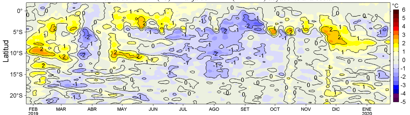
Figura 4. Variación promedio de las anomalías de la temperatura superficial del mar (TSM, °C) para una franja de 60 mn (~111 km) adyacente al litoral peruano para los últimos doce meses al 24 de enero de 2020. Datos: OSTIA-UKMO-L4-GLOB-v2.0 (UK Met. Office, 2012; Donlon et al, 2012) disponible en https://podaac.jpl.nasa.gov/dataset/OSTIA-UKMO-L4-GLOB-v2.0 . Las anomalías se calcularon con respecto al periodo 2007-2016. Procesamiento: LHFM/AFIOF/DGIOCC/IMARPE.
