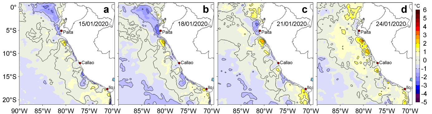
Figura 3. Anomalías de la temperatura superficial del mar (TSM, °C) para los días: a) 15, b) 18, c) 21 y d) 24 de enero de 2020. Las anomalías se calcularon respecto de la climatología para el periodo 2007-2016. Datos: OSTIA-UKMO-L4-GLOB-v2.0 (UK Met Office, 2012; Donlon et al, 2012). Procesamiento: LHFM/AFIOF/DGIOCC/IMARPE.
