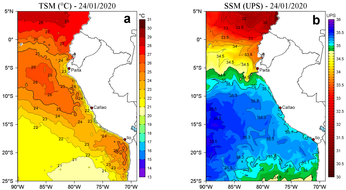
Figura 2. a) Temperatura superficial del mar (TSM, °C) y b) Salinidad superficial del mar (SSM, UPS), para el 24 de enero de 2020. Datos: OSTIA-UKMO-L4-GLOB-v2.0 (UK Met Office, 2012; Donlon et al, 2012) disponible en https://podaac.jpl.nasa.gov/dataset/OSTIA-UKMO-L4-GLOB-v2.0 para (a) y Hybrid Coordinate Ocean Model v. GOF3 3.1 (HYCOM; Halliwell et al., 1998; 2000; Bleck, 2001) para (b). Procesamiento: LHFM/AFIOF/DGIOCC/IMARPE.
