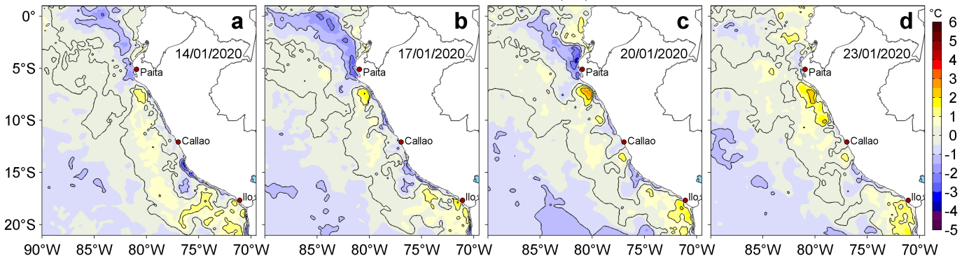
Figura 3. Anomalías de la temperatura superficial del mar (TSM, °C) para los días: a) 14, b) 17, c) 20 y d) 23 de enero de 2020. Las anomalías se calcularon respecto de la climatología para el periodo 2007-2016. Datos: OSTIA-UKMO-L4-GLOB-v2.0 (UK Met Office, 2012; Donlon et al, 2012). Procesamiento: LHF/AFIOF/DGIOCC/IMARPE.
