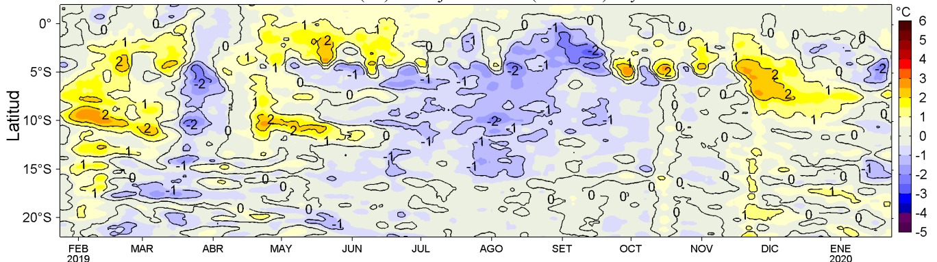
Figura 4. Variación promedio de las anomalías de la temperatura superficial del mar (TSM, °C) para una franja de 60 mn (~111 km) adyacente al litoral peruano para los últimos doce meses al 23 de enero de 2020. Datos: OSTIA-UKMO-L4-GLOB-v2.0 (UK Met. Office, 2012; Donlon et al, 2012) disponible en https://podaac.jpl.nasa.gov/dataset/OSTIA-UKMO-L4-GLOB-v2.0 . Las anomalías se calcularon con respecto al periodo 2007-2016. Procesamiento: LHF/AFIOF/DGIOCC/IMARPE.
