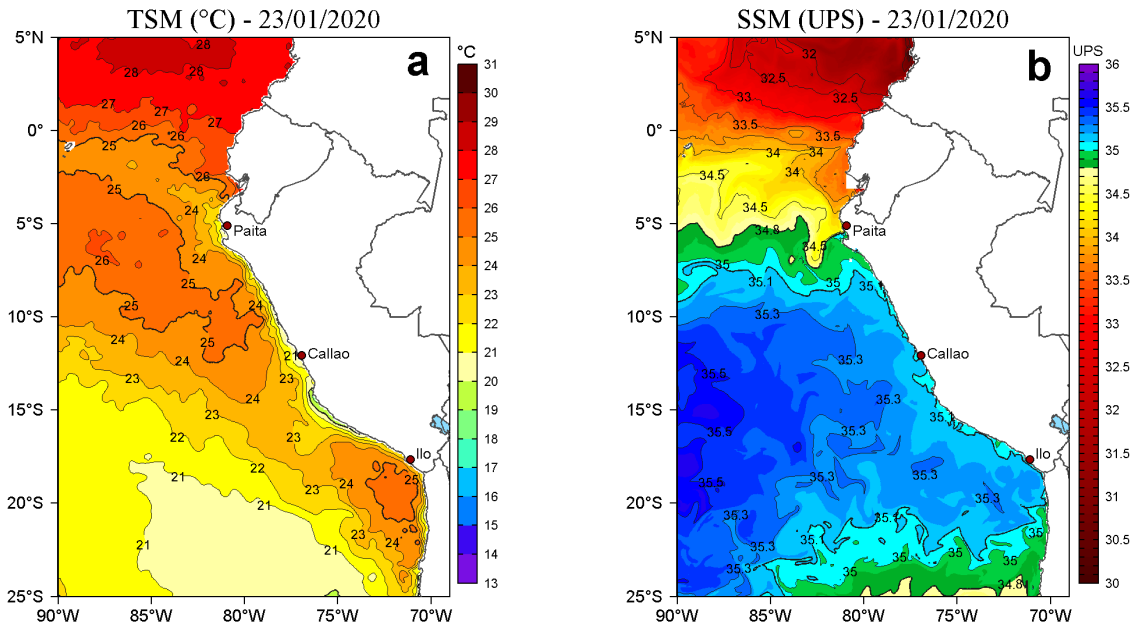
Figura 2. a) Temperatura superficial del mar (TSM, °C) y b) Salinidad superficial del mar (SSM, UPS), para el 23 de enero de 2020. Datos: OSTIA-UKMO-L4-GLOB-v2.0 (UK Met Office, 2012; Donlon et al, 2012) disponible en https://podaac.jpl.nasa.gov/dataset/OSTIA-UKMO-L4-GLOB-v2.0 para (a) y Hybrid Coordinate Ocean Model v. GOF5 3.1 (HYCOM; Halliwell et al., 1998; 2000; Bleck, 2001) para (b). Procesamiento: LHF/AFIOF/DGIOCC/IMARPE.
