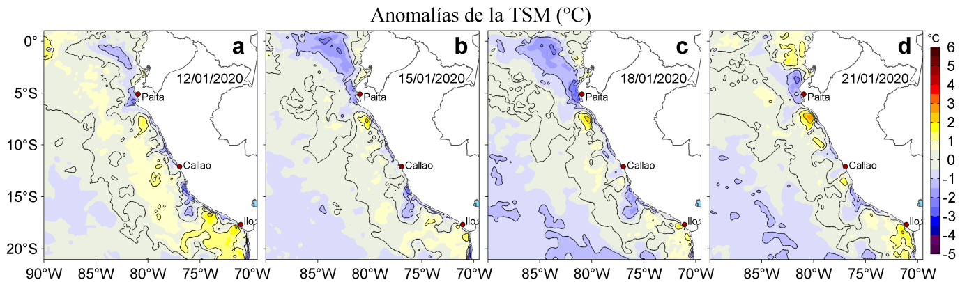
Figura 3. Anomalías de la temperatura superficial del mar (TSM, °C) para los días: a) 12, b) 15, c) 18 y d) 21 de enero de 2020. Las anomalías se calcularon respecto de la climatología para el periodo 2007-2016. Datos: OSTIA-UKMO-L4-GLOB-v2.0 (UK Met Office, 2012; Donlon et al, 2012). Procesamiento: LHFM/AFIOF/DGIOCC/IMARPE.
