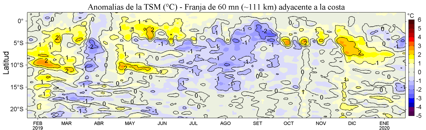
Figura 4. Variación promedio de las anomalías de la temperatura superficial del mar (TSM, °C) para una franja de 60 mn (~111 km) adyacente al litoral peruano para los últimos doce meses al 21 de enero de 2020. Datos: OSTIA-UKMO-L4-GLOB-v2.0 (UK Met. Office, 2012; Donlon et al, 2012) disponible en https://podaac.jpl.nasa.gov/dataset/OSTIA-UKMO-L4-GLOB-v2.0 . Las anomalías se calcularon con respecto al periodo 2007-2016. Procesamiento: LHFM/AFIOF/DGIOCC/IMARPE.
