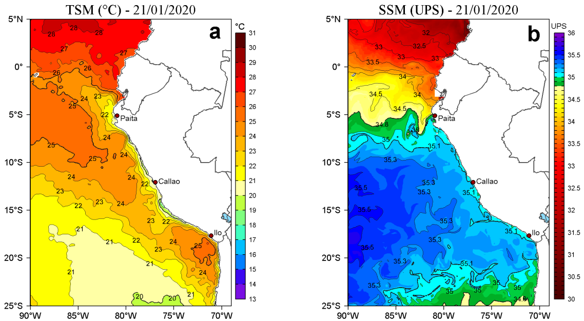
Figura 2. a) Temperatura superficial del mar (TSM, °C) y b) Salinidad superficial del mar (SSM, UPS), para el 21 de enero de 2020. Datos: OSTIA-UKMO-L4-GLOB-v2.0 (UK Met Office, 2012; Donlon et al, 2012) disponible en https://podaac.jpl.nasa.gov/dataset/OSTIA-UKMO-L4-GLOB-v2.0 para (a) y Hybrid Coordinate Ocean Model v. GOF3 3.1 (HYCOM; Halliwell et al., 1998; 2000; Bleck, 2001) para (b). Procesamiento: LHFM/AFIOF/DGIOCC/IMARPE.
