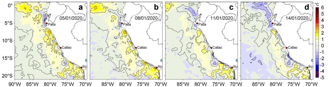
Figura 3. Anomalías de la temperatura superficial del mar (TSM, °C) para los días: a) 05, b) 08, c) 11 y d) 14 de enero de 2020. Las anomalías se calcularon respecto de la climatología para el periodo 2007-2016. Datos: OSTIA-UKMO-L4-GLOB-v2.0 (UK Met Office, 2012; Donlon et al, 2012). Procesamiento: LHF/AFIOF/DGIOCC/IMARPE.
