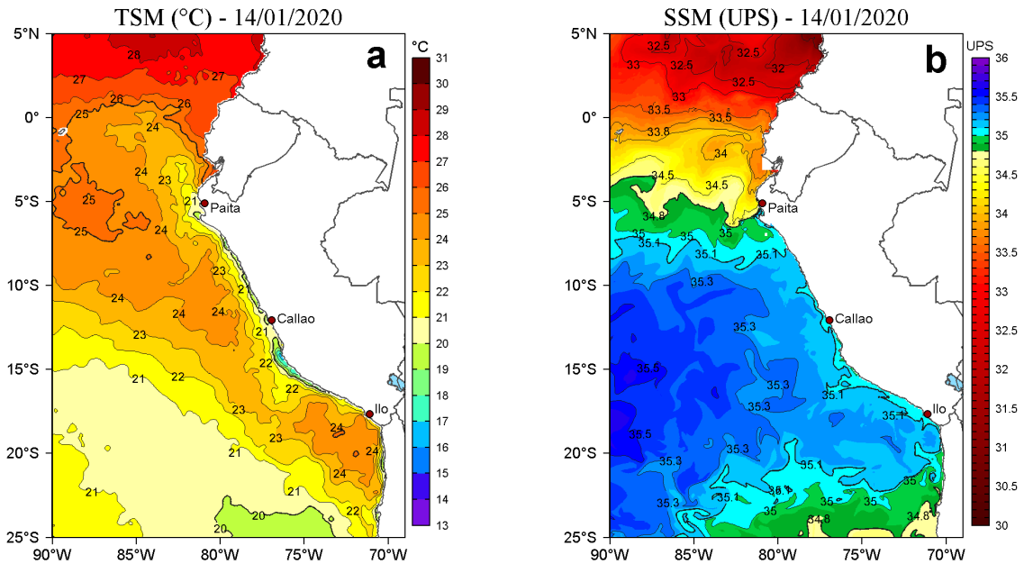
Figura 2. a) Temperatura superficial del mar (TSM, °C) y b) Salinidad superficial del mar (SSM, UPS), para el 14 de enero de 2020. Datos: OSTIA-UKMO-L4-GLOB-v2.0 (UK Met Office, 2012; Donlon et al, 2012) disponible en https://podaac.jpl.nasa.gov/dataset/OSTIA-UKMO-L4-GLOB-v2.0 para (a) y Hybrid Coordinate Ocean Model v. GOF3 3.1 (HYCOM; Halliwell et al., 1998; 2000; Bleck, 2001) para (b). Procesamiento: LHF/AFIOF/DGIOCC/IMARPE.
