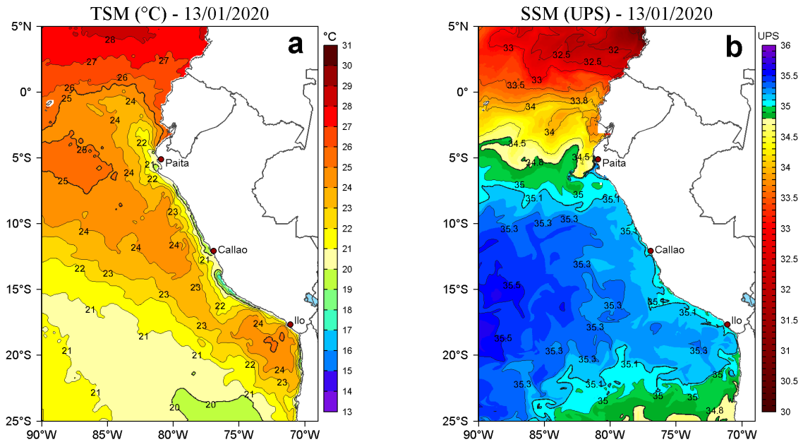
Figura 2. a) Temperatura superficial del mar (TSM, °C) y b) Salinidad superficial del mar (SSM, UPS), para el 13 de enero de 2020. Datos: OSTIA-UKMO-L4-GLOB-v2.0 (UK Met Office, 2012; Donlon et al, 2012) disponible en https://podaac.jpl.nasa.gov/dataset/OSTIA-UKMO-L4-GLOB-v2.0 para (a) y Hybrid Coordinate Ocean Model v. GOF5 3.1 (HYCOM; Halliwell et al., 1998; 2000; Bleck, 2001) para (b). Procesamiento: LHF/AFIOF/DGIOCC/IMARPE.
