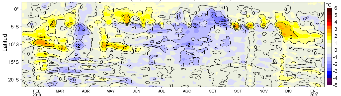
Figura 4. Variación promedio de las anomalías de la temperatura superficial del mar (TSM, °C) para una franja de 60 mn (~111 km) adyacente al litoral peruano para los últimos doce meses al 13 de enero de 2020. Datos: OSTIA-UKMO-L4-GLOB-v2.0 (UK Met. Office, 2012; Donlon et al, 2012) disponible en https://podaac.jpl.nasa.gov/dataset/OSTIA-UKMO-L4-GLOB-v2.0 . Las anomalías se calcularon con respecto al periodo 2007-2016. Procesamiento: LHF/AFIOF/DGIOCC/IMARPE.
