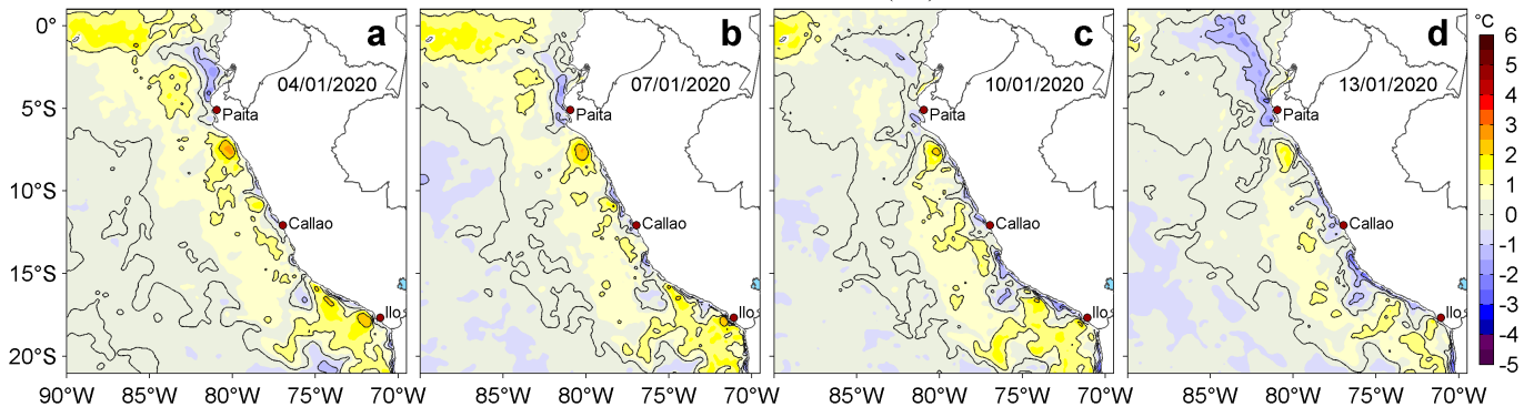
Figura 3. Anomalías de la temperatura superficial del mar (TSM, °C) para los días: a) 04, b) 07, c) 10 y d) 13 de enero de 2020. Las anomalías se calcularon respecto de la climatología para el periodo 2007-2016. Datos: OSTIA-UKMO-L4-GLOB-v2.0 (UK Met Office, 2012; Donlon et al, 2012). Procesamiento: LHF/AFIOF/DGIOCC/IMARPE.
