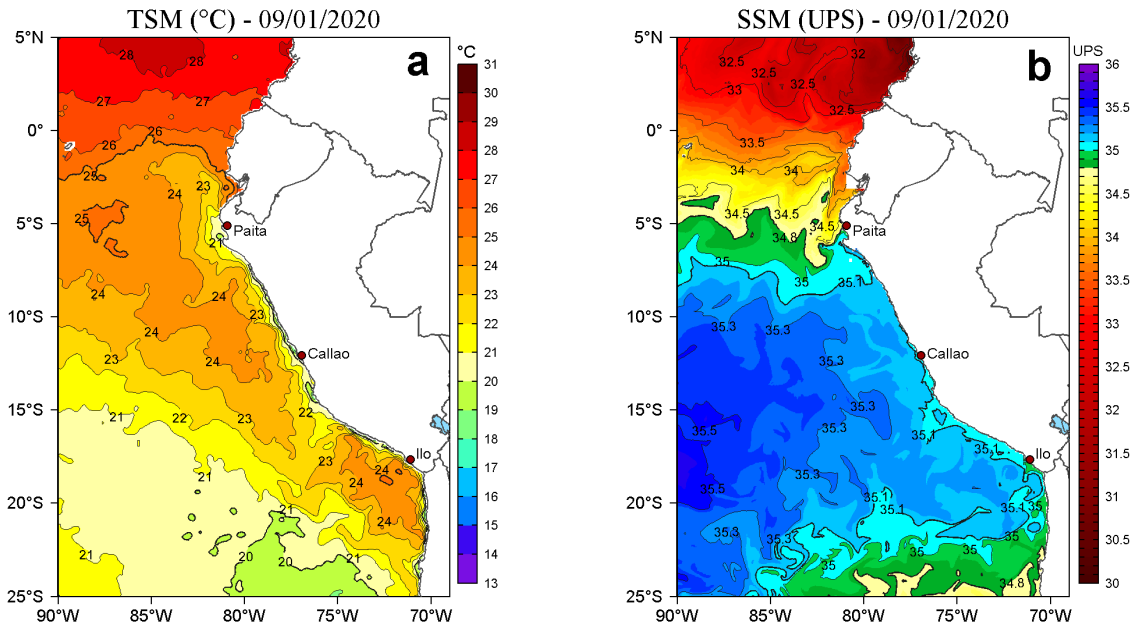
Figura 2. a) Temperatura superficial del mar (TSM, °C) y b) Salinidad superficial del mar (SSM, UPS), para el 09 de enero de 2020. Datos: OSTIA-UKMO-L4-GLOB-v2.0 (UK Met Office, 2012; Donlon et al, 2012) disponible en https://podaac.jpl.nasa.gov/dataset/OSTIA-UKMO-L4-GLOB-v2.0 para (a) y Hybrid Coordinate Ocean Model v. GOF3.1 (HYCOM; Halliwell et al., 1998; 2000; Bleck, 2001) para (b). Procesamiento: LHFM/AFIOF/DGIOCC/IMARPE.
