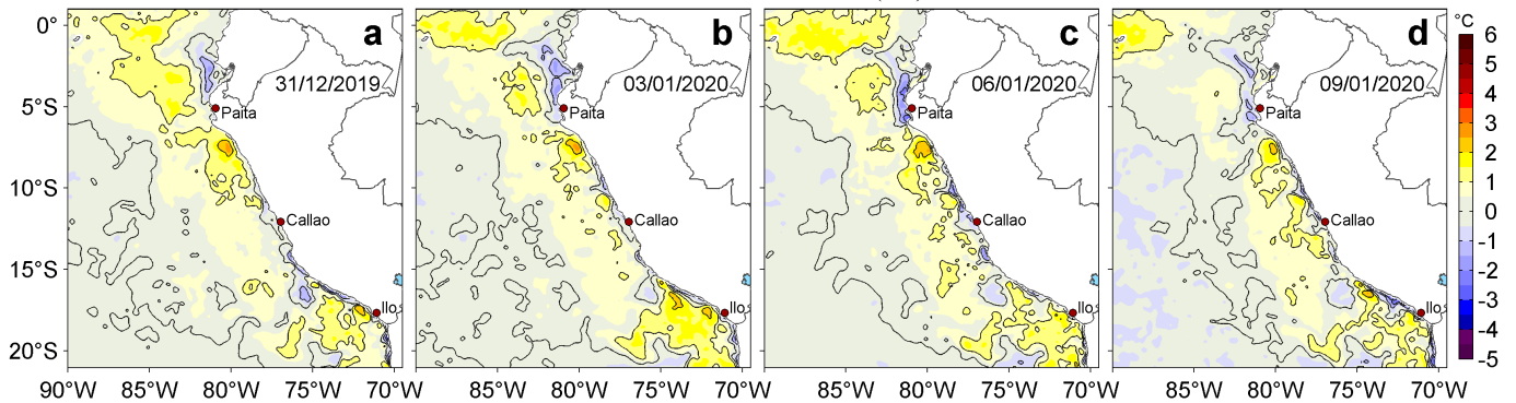
Figura 3. Anomalías de la temperatura superficial del mar (TSM, °C) para los días: a) 31 de diciembre de 2019, b) 03, c) 06 y d) 09 de enero de 2020. Las anomalías se calcularon respecto de la climatología para el periodo 2007-2016. Datos: OSTIA-UKMO-L4-GLOB-v2.0 (UK Met Office, 2012; Donlon et al, 2012). Procesamiento: LHFM/AFIOF/DGIOCC/IMARPE.
