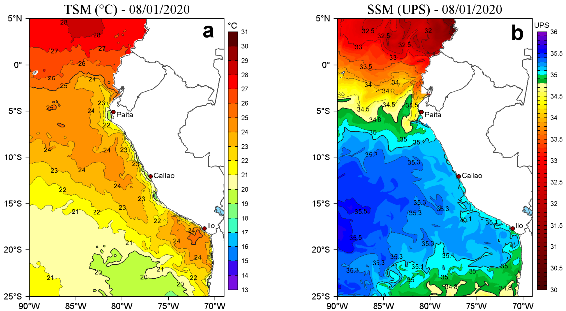
Figura 2. a) Temperatura superficial del mar (TSM, °C) y b) Salinidad superficial del mar (SSM, UPS), para el 08 de enero de 2020. Datos: OSTIA-UKMO-L4-GLOB-v2.0 (UK Met Office, 2012; Donlon et al, 2012) disponible en https://podaac.jpl.nasa.gov/dataset/OSTIA-UKMO-L4-GLOB-v2.0 para (a) y Hybrid Coordinate Ocean Model v. GOF3 3.1 (HYCOM; Halliwell et al., 1998; 2000; Bleck, 2001) para (b). Procesamiento: LHFM/AFIOF/DGIOCC/IMARPE.
