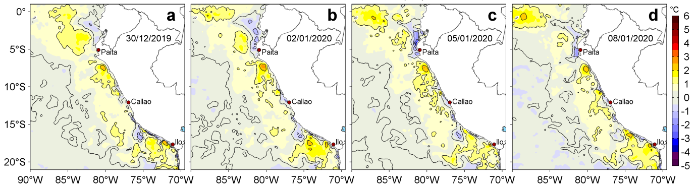
Figura 3. Anomalías de la temperatura superficial del mar (TSM, °C) para los días: a) 30 de diciembre de 2019, b) 02, c) 05 y d) 08 de enero de 2020. Las anomalías se calcularon respecto de la climatología para el periodo 2007-2016. Datos: OSTIA-UKMO-L4-GLOB-v2.0 (UK Met Office, 2012; Donlon et al, 2012). Procesamiento: LHFM/AFIOF/DGIOCC/IMARPE.
