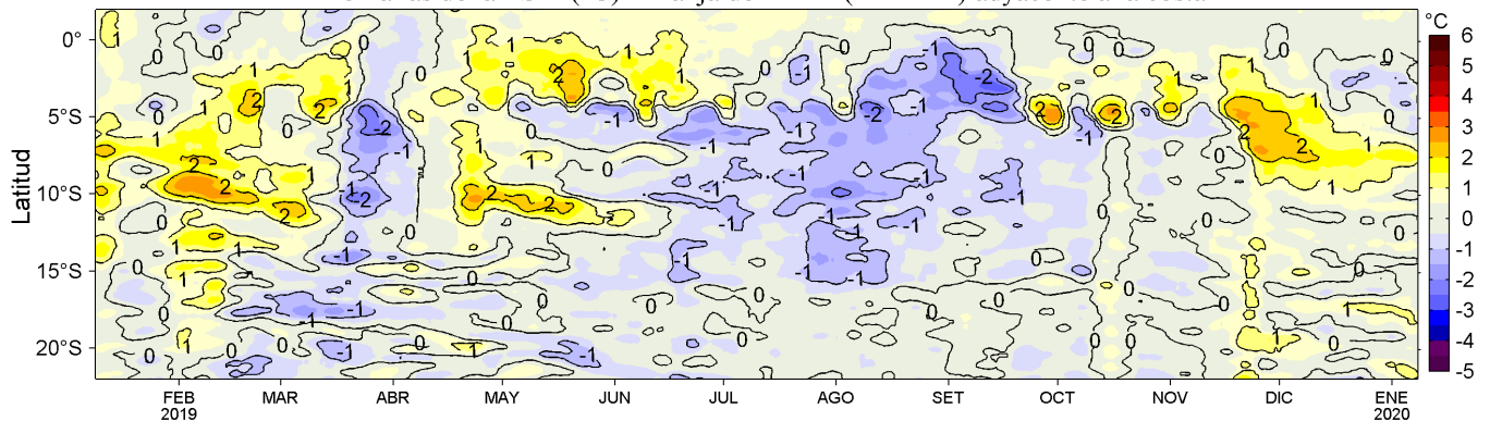
Figura 4. Variación promedio de las anomalías de la temperatura superficial del mar (TSM, °C) para una franja de 60 mn (~111 km) adyacente al litoral peruano para los últimos doce meses al 08 de enero de 2020. Datos: OSTIA-UKMO-L4-GLOB-v2.0 (UK Met. Office, 2012; Donlon et al, 2012) disponible en https://podaac.jpl.nasa.gov/dataset/OSTIA-UKMO-L4-GLOB-v2.0 . Las anomalías se calcularon con respecto al periodo 2007-2016. Procesamiento: LHFM/AFIOF/DGIOCC/IMARPE.
