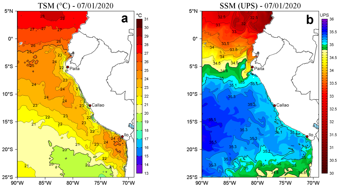
Figura 2. a) Temperatura superficial del mar (TSM, °C) y b) Salinidad superficial del mar (SSM, UPS), para el 07 de enero de 2020. Datos: OSTIA-UKMO-L4-GLOB-v2.0 (UK Met Office, 2012; Donlon et al, 2012) disponible en https://podaac.jpl.nasa.gov/dataset/OSTIA-UKMO-L4-GLOB-v2.0 para (a) y Hybrid Coordinate Ocean Model v. GOF3.1 (HYCOM; Halliwell et al., 1998; 2000; Bleck, 2001) para (b). Procesamiento: LHFM/AFIOF/DGIOCC/IMARPE.
