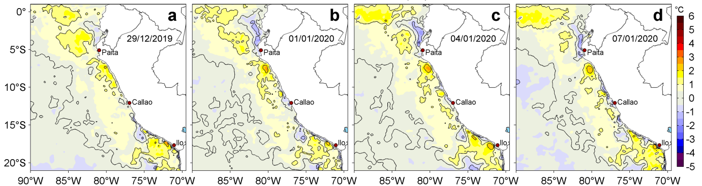
Figura 3. Anomalías de la temperatura superficial del mar (TSM, °C) para los días: a) 29 de diciembre de 2019, b) 01, c) 04 y d) 07 de enero de 2020. Las anomalías se calcularon respecto de la climatología para el periodo 2007-2016. Datos: OSTIA-UKMO-L4-GLOB-v2.0 (UK Met Office, 2012; Donlon et al, 2012). Procesamiento: LHFM/AFIOF/DGIOCC/IMARPE.
