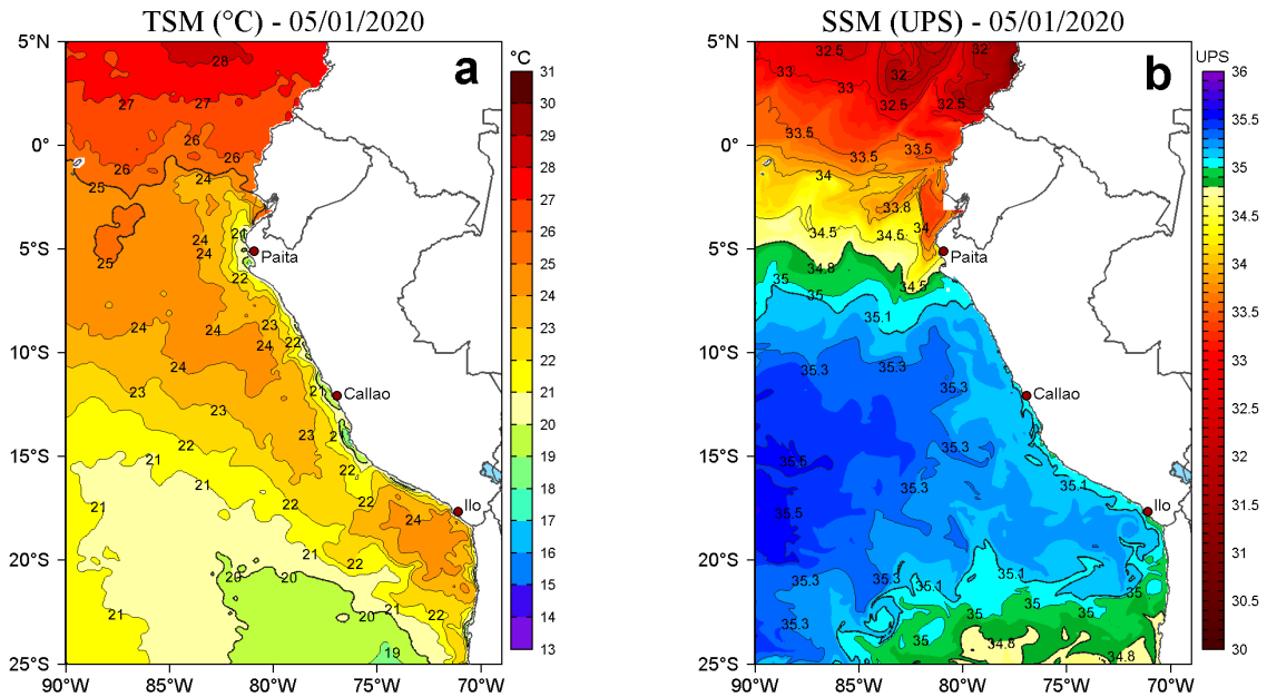
Figura 2. a) Temperatura superficial del mar (TSM, °C) y b) Salinidad superficial del mar (SSM, UPS), para el 05 de enero de 2020. Datos: OSTIA-UKMO-L4-GLOB-v2.0 (UK Met Office, 2012; Donlon et al, 2012) disponible en https://podaac.jpl.nasa.gov/dataset/OSTIA-UKMO-L4-GLOB-v2.0 para (a) y Hybrid Coordinate Ocean Model v. GOF3.1 (HYCOM; Halliwell et al., 1998; 2000; Bleck, 2001) para (b). Procesamiento: LHFM/AFIOF/DGIOCC/IMARPE.
