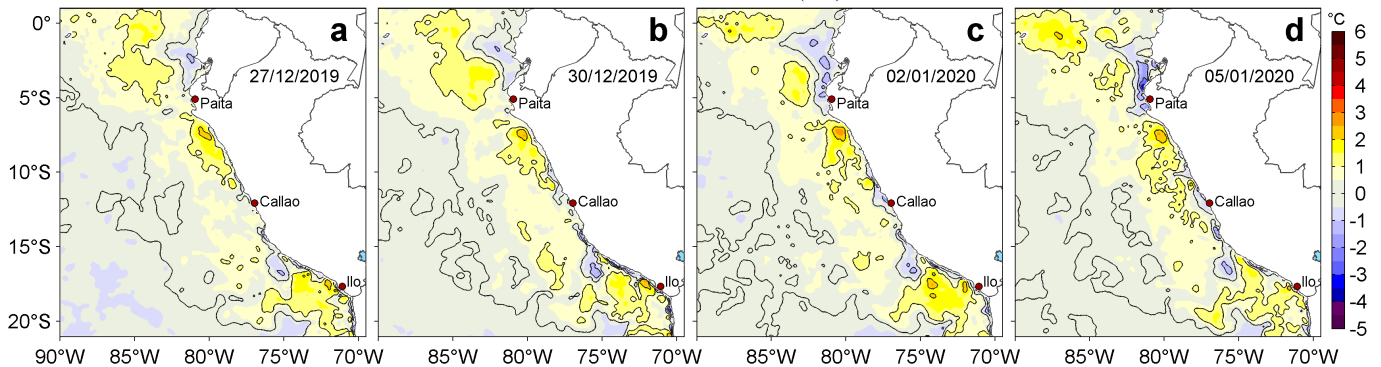
Figura 3. Anomalías de la temperatura superficial del mar (TSM, °C) para los días: a) 27 y b) 30 de diciembre de 2019, c) 02 y d) 05 de enero de 2020. Las anomalías se calcularon respecto de la climatología para el periodo 2007-2016. Datos: OSTIA-UKMO-L4-GLOB-v2.0 (UK Met Office, 2012; Donlon et al, 2012). Procesamiento: LHFM/AFIOF/DGIOCC/IMARPE.
