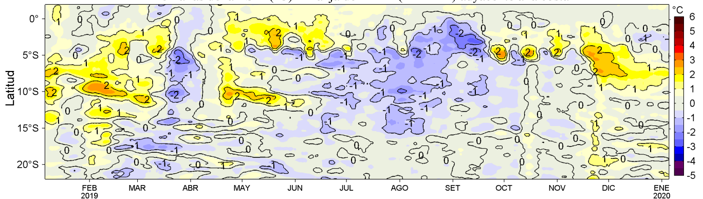
Figura 4. Variación promedio de las anomalías de la temperatura superficial del mar (TSM, °C) para una franja de 60 mn (~111 km) adyacente al litoral peruano para los últimos doce meses al 05 de enero de 2020. Datos: OSTIA-UKMO-L4-GLOB-v2.0 (UK Met. Office, 2012; Donlon et al, 2012) disponible en https://podaac.jpl.nasa.gov/dataset/OSTIA-UKMO-L4-GLOB-v2.0 . Las anomalías se calcularon con respecto al periodo 2007-2016. Procesamiento: LHFM/AFIOF/DGIOCC/IMARPE.
