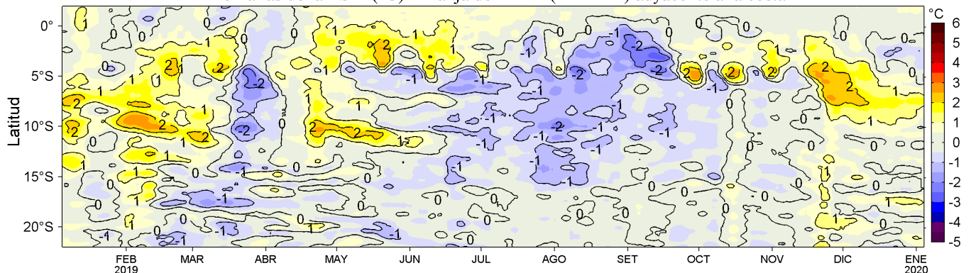
Figura 4. Variación promedio de las anomalías de la temperatura superficial del mar (TSM, °C) para una franja de 60 mn (~111 km) adyacente al litoral peruano para los últimos doce meses al 04 de enero de 2020. Datos: OSTIA-UKMO-L4-GLOB-v2.0 (UK Met. Office, 2012; Donlon et al, 2012) disponible en https://podaac.jpl.nasa.gov/dataset/OSTIA-UKMO-L4-GLOB-v2.0 . Las anomalías se calcularon con respecto al periodo 2007-2016. Procesamiento: LHFM/AFIOF/DGIOCC/IMARPE.
