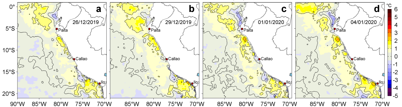
Figura 3. Anomalías de la temperatura superficial del mar (TSM, °C) para los días: a) 26 y b) 29 de diciembre de 2019, c) 01 y d) 04 de enero de 2020. Las anomalías se calcularon respecto de la climatología para el periodo 2007-2016. Datos: OSTIA-UKMO-L4-GLOB-v2.0 (UK Met Office, 2012; Donlon et al, 2012). Procesamiento: LHFM/AFIOF/DGIOCC/IMARPE.
