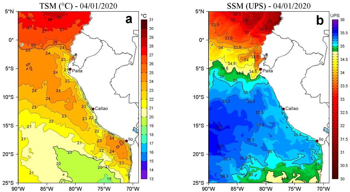
Figura 2. a) Temperatura superficial del mar (TSM, °C) y b) Salinidad superficial del mar (SSM, UPS), para el 04 de enero de 2020. Datos: OSTIA-UKMO-L4-GLOB-v2.0 (UK Met Office, 2012; Donlon et al, 2012) disponible en https://podaac.jpl.nasa.gov/dataset/OSTIA-UKMO-L4-GLOB-v2.0 para (a) y Hybrid Coordinate Ocean Model v. GOF3 3.1 (HYCOM; Halliwell et al., 1998; 2000; Bleck, 2001) para (b). Procesamiento: LHFM/AFIOF/DGIOCC/IMARPE.
