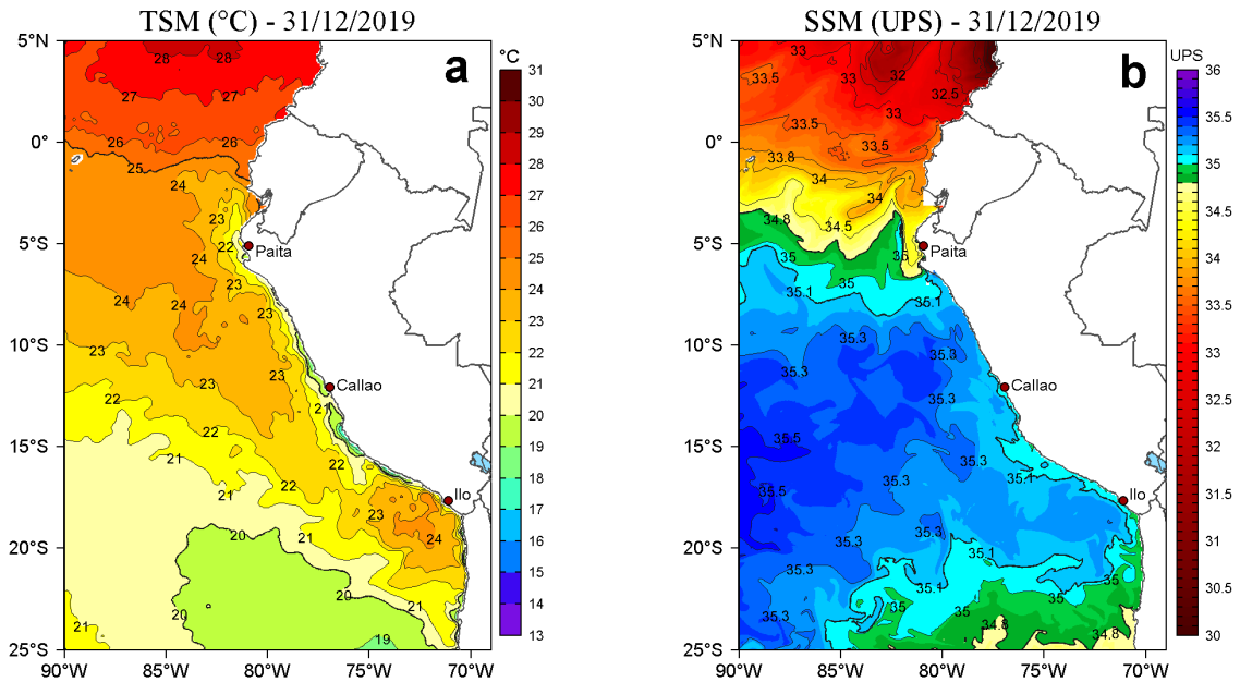
Figura 2. a) Temperatura superficial del mar (TSM, °C) y b) Salinidad superficial del mar (SSM, UPS), para el 31 de diciembre de 2019. Datos: OSTIA-UKMO-L4-GLOB-v2.0 (UK Met Office, 2012; Donlon et al, 2012) disponible en https://podaac.jpl.nasa.gov/dataset/OSTIA-UKMO-L4-GLOB-v2.0 para (a) y Hybrid Coordinate Ocean Model v. GOFS 3.1 (HYCOM; Halliwell et al., 1998; 2000; Bleck, 2001) para (b). Procesamiento: LHF/AFIOF/DGIOCC/IMARPE.
