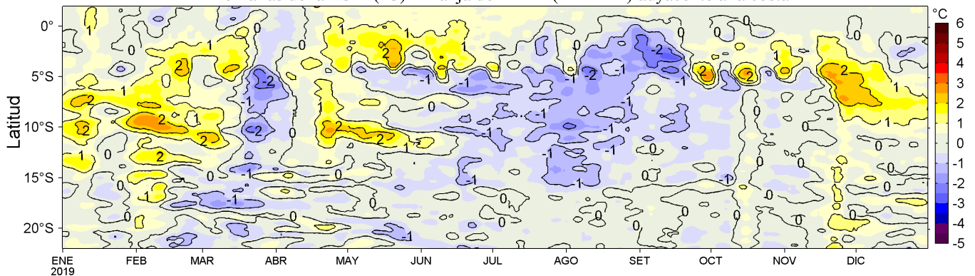
Figura 4. Variación promedio de las anomalías de la temperatura superficial del mar (TSM, °C) para una franja de 60 mn (~111 km) adyacente al litoral peruano para los últimos doce meses al 31 de diciembre de 2019. Datos: OSTIA-UKMO-L4-GLOB-v2.0 (UK Met. Office, 2012; Donlon et al, 2012) disponible en https://podaac.jpl.nasa.gov/dataset/OSTIA-UKMO-L4-GLOB-v2.0 . Las anomalías se calcularon con respecto al periodo 2007-2016. Procesamiento: LHF/AFIOF/DGIOCC/IMARPE.
