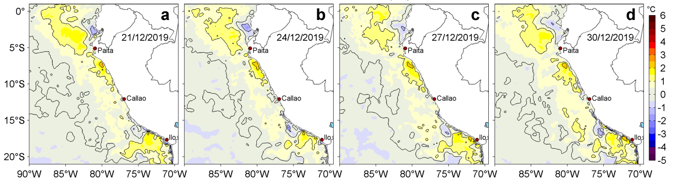
Figura 3. Anomalías de la temperatura superficial del mar (TSM, °C) para los días: a) 21, b) 24, c) 27 y d) 30 de diciembre de 2019. Las anomalías se calcularon respecto de la climatología para el periodo 2007-2016. Datos: OSTIA-UKMO-L4-GLOB-v2.0 (UK Met Office, 2012; Donlon et al, 2012). Procesamiento: LHF/AFIOF/DGIOCC/IMARPE.
