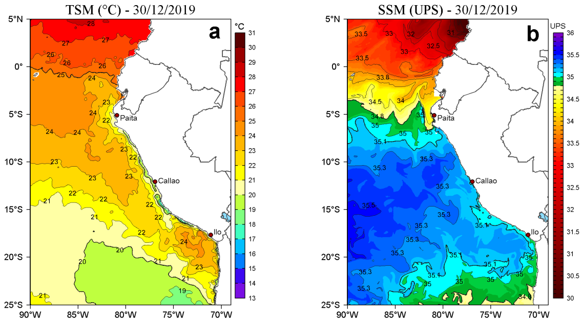
Figura 2. a) Temperatura superficial del mar (TSM, °C) y b) Salinidad superficial del mar (SSM, UPS), para el 30 de diciembre de 2019. Datos: OSTIA-UKMO-L4-GLOB-v2.0 (UK Met Office, 2012; Donlon et al, 2012) disponible en https://podaac.jpl.nasa.gov/dataset/OSTIA-UKMO-L4-GLOB-v2.0 para (a) y Hybrid Coordinate Ocean Model v. GOFS 3.1 (HYCOM; Halliwell et al., 1998; 2000; Bleck, 2001) para (b). Procesamiento: LHF/AFIOF/DGIOCC/IMARPE.
