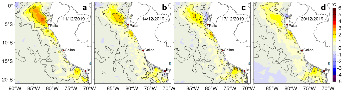
Figura 3. Anomalías de la temperatura superficial del mar (TSM, °C) para los días: a) 11, b) 14, c) 17 y d) 20 de diciembre de 2019. Las anomalías se calcularon respecto de la climatología para el periodo 2007-2016. Datos: OSTIA-UKMO-L4-GLOB-v2.0 (UK Met Office, 2012; Donlon et al, 2012). Procesamiento: LHF/AFIOF/DGIOCC/IMARPE.
