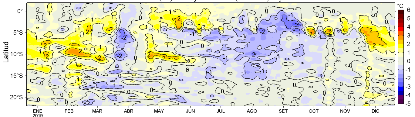
Figura 4. Variación promedio de las anomalías de la temperatura superficial del mar (TSM, °C) para una franja de 60 mn (~111 km) adyacente al litoral peruano para los últimos doce meses al 20 de diciembre de 2019. Datos: OSTIA-UKMO-L4-GLOB-v2.0 (UK Met. Office, 2012; Donlon et al, 2012) disponible en https://podaac.jpl.nasa.gov/dataset/OSTIA-UKMO-L4-GLOB-v2.0 . Las anomalías se calcularon con respecto al periodo 2007-2016. Procesamiento: LHF/AFIOF/DGIOCC/IMARPE.
