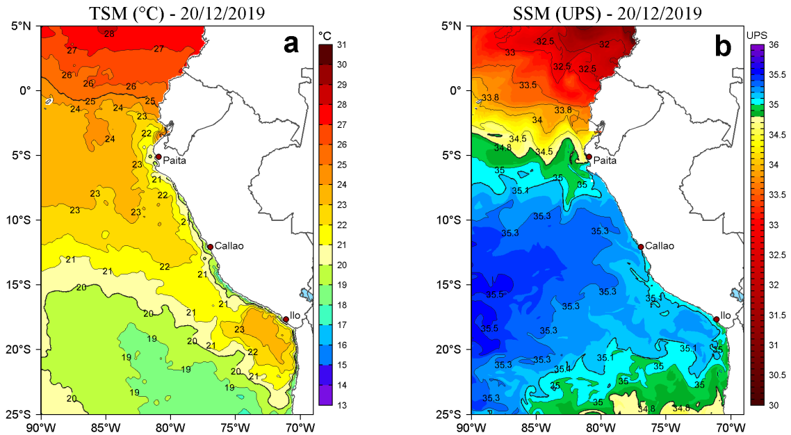
Figura 2. a) Temperatura superficial del mar (TSM, °C) y b) Salinidad superficial del mar (SSM, UPS), para el 20 de diciembre de 2019. Datos: OSTIA-UKMO-L4-GLOB-v2.0 (UK Met Office, 2012; Donlon et al, 2012) disponible en https://podaac.jpl.nasa.gov/dataset/OSTIA-UKMO-L4-GLOB-v2.0 para (a) y Hybrid Coordinate Ocean Model v. GOFS 3.1 (HYCOM; Halliwell et al., 1998; 2000; Bleck, 2001) para (b). Procesamiento: LHF/AFIOF/DGIOCC/IMARPE.
