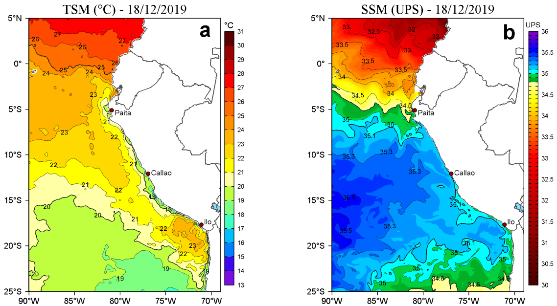
Figura 2. a) Temperatura superficial del mar (TSM, °C) y b) Salinidad superficial del mar (SSM, UPS), para el 18 de diciembre de 2019. Datos: OSTIA-UKMO-L4-GLOB-v2.0 (UK Met Office, 2012; Donlon et al, 2012) disponible en https://podaac.jpl.nasa.gov/dataset/OSTIA-UKMO-L4-GLOB-v2.0 para (a) y Hybrid Coordinate Ocean Model v. GOFS 3.1 (HYCOM; Halliwell et al., 1998; 2000; Bleck, 2001) para (b). Procesamiento: LHF/AFIOF/DGIOCC/IMARPE.
