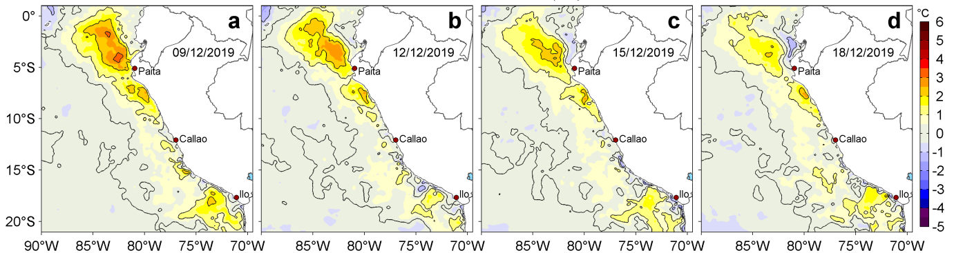
Figura 3. Anomalías de la temperatura superficial del mar (TSM, °C) para los días: a) 09, b) 12, c) 15 y d) 18 de diciembre de 2019. Las anomalías se calcularon respecto de la climatología para el periodo 2007-2016. Datos: OSTIA-UKMO-L4-GLOB-v2.0 (UK Met Office, 2012; Donlon et al, 2012). Procesamiento: LHF/AFIOF/DGIOCC/IMARPE.
