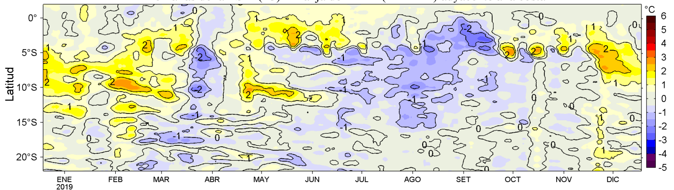
Figura 4. Variación promedio de las anomalías de la temperatura superficial del mar (TSM, °C) para una franja de 60 mn (~111 km) adyacente al litoral peruano para los últimos doce meses al 18 de diciembre de 2019. Datos: OSTIA-UKMO-L4-GLOB-v2.0 (UK Met. Office, 2012; Donlon et al, 2012) disponible en https://podaac.jpl.nasa.gov/dataset/OSTIA-UKMO-L4-GLOB-v2.0 . Las anomalías se calcularon con respecto al periodo 2007-2016. Procesamiento: LHF/AFIOF/DGIOCC/IMARPE.
