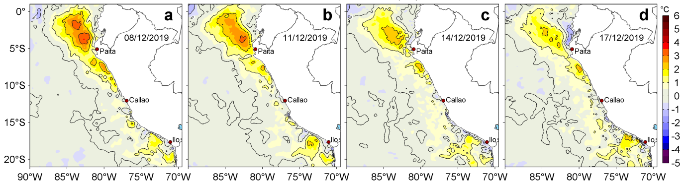
Figura 3. Anomalías de la temperatura superficial del mar (TSM, °C) para los días: a) 08, b) 11, c) 14 y d) 17 de diciembre de 2019. Las anomalías se calcularon respecto de la climatología para el periodo 2007-2016. Datos: OSTIA-UKMO-L4-GLOB-v2.0 (UK Met Office, 2012; Donlon et al, 2012). Procesamiento: LHF/AFIOF/DGIOCC/IMARPE.
