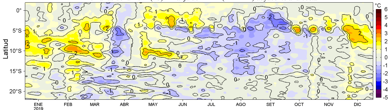
Figura 4. Variación promedio de las anomalías de la temperatura superficial del mar (TSM, °C) para una franja de 60 mn (~111 km) adyacente al litoral peruano para los últimos doce meses al 17 de diciembre de 2019. Datos: OSTIA-UKMO-L4-GLOB-v2.0 (UK Met. Office, 2012; Donlon et al, 2012) disponible en https://podaac.jpl.nasa.gov/dataset/OSTIA-UKMO-L4-GLOB-v2.0 . Las anomalías se calcularon con respecto al periodo 2007-2016. Procesamiento: LHF/AFIOF/DGIOCC/IMARPE.
