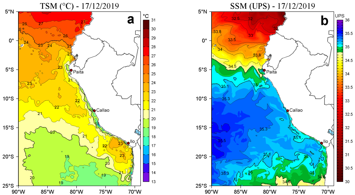
Figura 2. a) Temperatura superficial del mar (TSM, °C) y b) Salinidad superficial del mar (SSM, UPS), para el 17 de diciembre de 2019. Datos: OSTIA-UKMO-L4-GLOB-v2.0 (UK Met Office, 2012; Donlon et al, 2012) disponible en https://podaac.jpl.nasa.gov/dataset/OSTIA-UKMO-L4-GLOB-v2.0 para (a) y Hybrid Coordinate Ocean Model v. GOFS 3.1 (HYCOM; Halliwell et al., 1998; 2000; Bleck, 2001) para (b). Procesamiento: LHF/AFIOF/DGIOCC/IMARPE.
