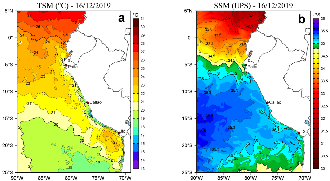
Figura 2. a) Temperatura superficial del mar (TSM, °C) y b) Salinidad superficial del mar (SSM, UPS), para el 16 de diciembre de 2019. Datos: OSTIA-UKMO-L4-GLOB-v2.0 (UK Met Office, 2012; Donlon et al, 2012) disponible en https://podaac.jpl.nasa.gov/dataset/OSTIA-UKMO-L4-GLOB-v2.0 para (a) y Hybrid Coordinate Ocean Model v. GOFS 3.1 (HYCOM; Halliwell et al., 1998; 2000; Bleck, 2001) para (b). Procesamiento: LHF/AFIOF/DGIOCC/IMARPE.
