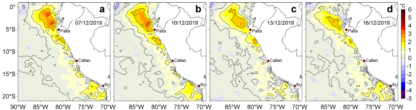
Figura 3. Anomalías de la temperatura superficial del mar (TSM, °C) para los días: a) 07, b) 10, c) 13 y d) 16 de diciembre de 2019. Las anomalías se calcularon respecto de la climatología para el periodo 2007-2016. Datos: OSTIA-UKMO-L4-GLOB-v2.0 (UK Met Office, 2012; Donlon et al, 2012). Procesamiento: LHF/AFIOF/DGIOCC/IMARPE.
