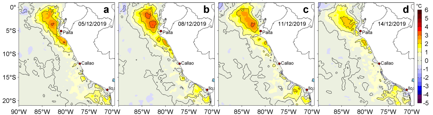
Figura 3. Anomalías de la temperatura superficial del mar (TSM, °C) para los días: a) 05, b) 08, c) 11 y d) 14 de diciembre de 2019. Las anomalías se calcularon respecto de la climatología para el periodo 2007-2016. Datos: OSTIA-UKMO-L4-GLOB-v2.0 (UK Met Office, 2012; Donlon et al, 2012). Procesamiento: LHF/AFIOF/DGIOCC/IMARPE.
