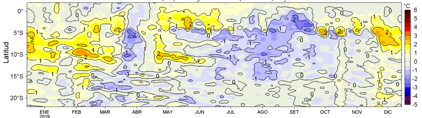
Figura 4. Variación promedio de las anomalías de la temperatura superficial del mar (TSM, °C) para una franja de 60 mn (~111 km) adyacente al litoral peruano para los últimos doce meses al 14 de diciembre de 2019. Datos: OSTIA-UKMO-L4-GLOB-v2.0 (UK Met. Office, 2012; Donlon et al, 2012) disponible en https://podaac.jpl.nasa.gov/dataset/OSTIA-UKMO-L4-GLOB-v2.0 . Las anomalías se calcularon con respecto al periodo 2007-2016. Procesamiento: LHF/AFIOF/DGIOCC/IMARPE.
