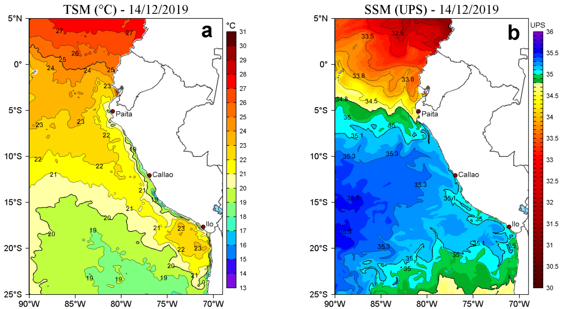
Figura 2. a) Temperatura superficial del mar (TSM, °C) y b) Salinidad superficial del mar (SSM, UPS), para el 14 de diciembre de 2019. Datos: OSTIA-UKMO-L4-GLOB-v2.0 (UK Met Office, 2012; Donlon et al, 2012) disponible en https://podaac.jpl.nasa.gov/dataset/OSTIA-UKMO-L4-GLOB-v2.0 para (a) y Hybrid Coordinate Ocean Model v. GOFS 3.1 (HYCOM; Halliwell et al., 1998; 2000; Bleck, 2001) para (b). Procesamiento: LHF/AFIOF/DGIOCC/IMARPE.
