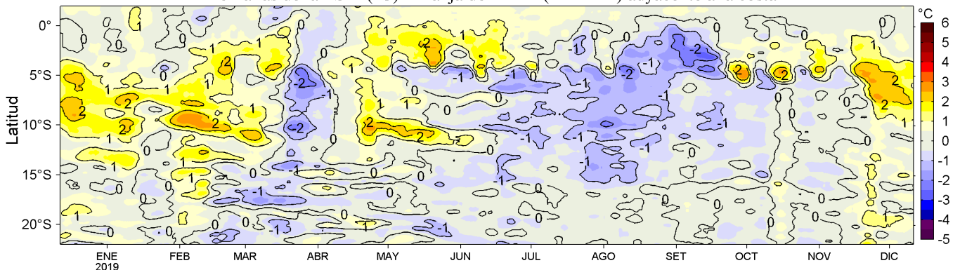
Figura 4. Variación promedio de las anomalías de la temperatura superficial del mar (TSM, °C) para una franja de 60 mn (~111 km) adyacente al litoral peruano para los últimos doce meses al 11 de diciembre de 2019. Datos: OSTIA-UKMO-L4-GLOB-v2.0 (UK Met. Office, 2012; Donlon et al, 2012) disponible en https://podaac.jpl.nasa.gov/dataset/OSTIA-UKMO-L4-GLOB-v2.0 . Las anomalías se calcularon con respecto al periodo 2007-2016. Procesamiento: LHF/AFIOF/DGIOCC/IMARPE.
