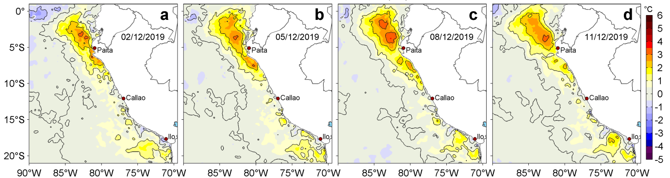
Figura 3. Anomalías de la temperatura superficial del mar (TSM, °C) para los días: a) 02, b) 05, c) 08 y d) 11 de diciembre de 2019. Las anomalías se calcularon respecto de la climatología para el periodo 2007-2016. Datos: OSTIA-UKMO-L4-GLOB-v2.0 (UK Met Office, 2012; Donlon et al, 2012). Procesamiento: LHF/AFIOF/DGIOCC/IMARPE.
