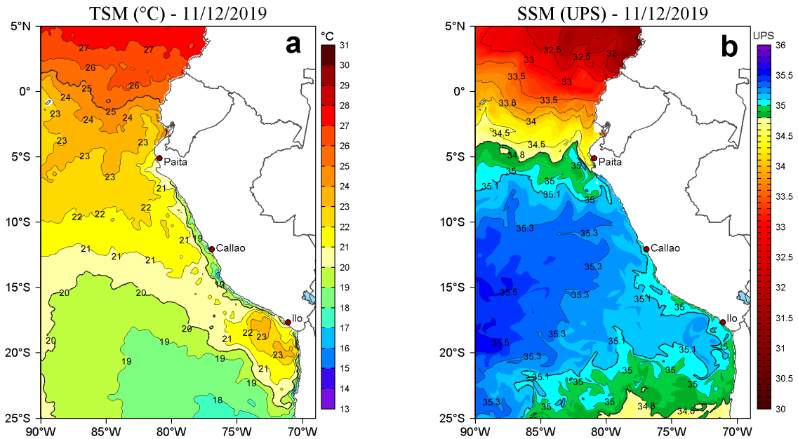
Figura 2. a) Temperatura superficial del mar (TSM, °C) y b) Salinidad superficial del mar (SSM, UPS), para el 11 de diciembre de 2019. Datos: OSTIA-UKMO-L4-GLOB-v2.0 (UK Met Office, 2012; Donlon et al, 2012) disponible en https://podaac.jpl.nasa.gov/dataset/OSTIA-UKMO-L4-GLOB-v2.0 para (a) y Hybrid Coordinate Ocean Model v. GOFS 3.1 (HYCOM; Halliwell et al., 1998; 2000; Bleck, 2001) para (b). Procesamiento: LHF/AFIOF/DGIOCC/IMARPE.
