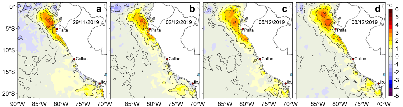
Figura 3. Anomalías de la temperatura superficial del mar (TSM, °C) para los días: a) 29 de noviembre, b) 02, c) 05 y d) 08 de diciembre de 2019. Las anomalías se calcularon respecto de la climatología para el periodo 2007-2016. Datos: OSTIA-UKMO-L4-GLOB-v2.0 (UK Met Office, 2012; Donlon et al, 2012). Procesamiento: LHF/AFIOF/DGIOCC/IMARPE.
