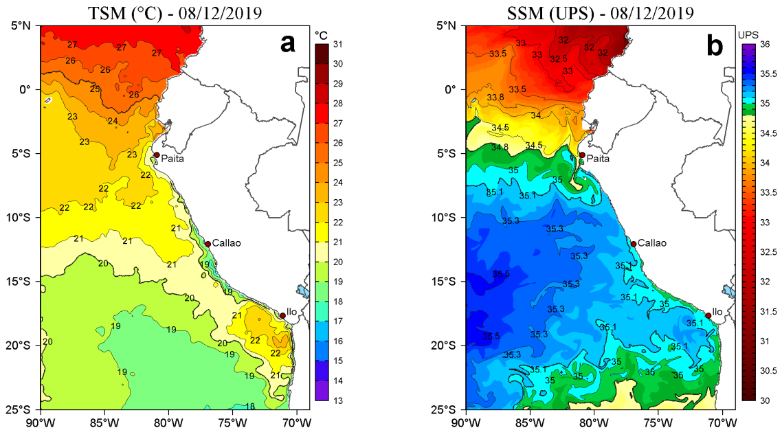
Figura 2. a) Temperatura superficial del mar (TSM, °C) y b) Salinidad superficial del mar (SSM, UPS), para el 08 de diciembre de 2019. Datos: OSTIA-UKMO-L4-GLOB-v2.0 (UK Met Office, 2012; Donlon et al, 2012) disponible en https://podaac.jpl.nasa.gov/dataset/OSTIA-UKMO-L4-GLOB-v2.0 para (a) y Hybrid Coordinate Ocean Model v. GOFS 3.1 (HYCOM; Halliwell et al., 1998; 2000; Bleck, 2001) para (b). Procesamiento: LHF/AFIOF/DGIOCC/IMARPE.
