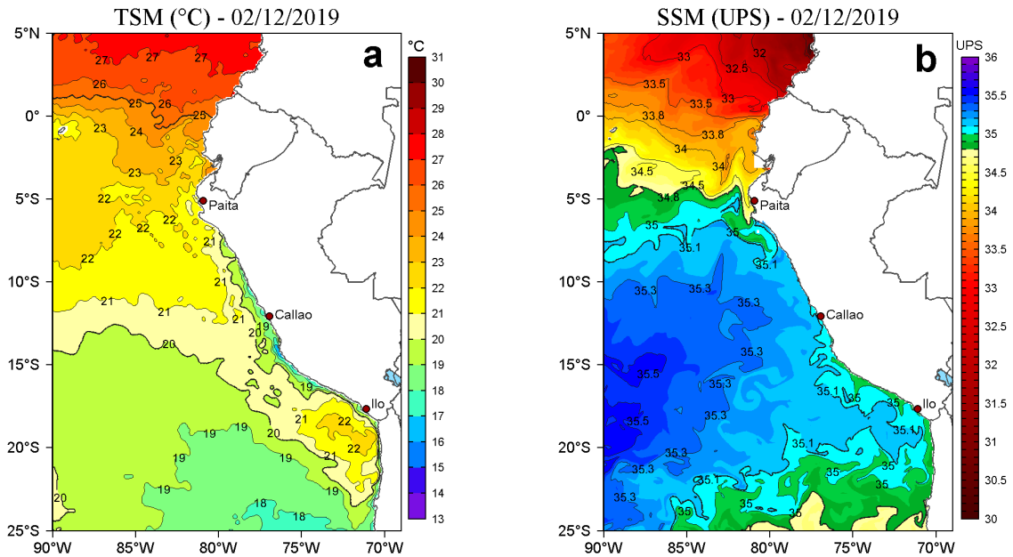
Figura 2. a) Temperatura superficial del mar (TSM, °C) y b) Salinidad superficial del mar (SSM, UPS), para el 02 de diciembre de 2019. Datos: OSTIA-UKMO-L4-GLOB-v2.0 (UK Met Office, 2012; Donlon et al, 2012) disponible en https://podaac.jpl.nasa.gov/dataset/OSTIA-UKMO-L4-GLOB-v2.0 para (a) y Hybrid Coordinate Ocean Model v. GOFS 3.1 (HYCOM; Halliwell et al., 1998; 2000; Bleck, 2001) para (b). Procesamiento: LHF/AFIOF/DGIOCC/IMARPE.
