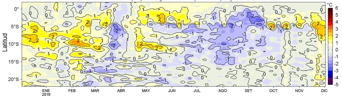
Figura 4. Variación promedio de las anomalías de la temperatura superficial del mar (TSM, °C) para una franja de 60 mn (~111 km) adyacente al litoral peruano para los últimos doce meses al 02 de diciembre de 2019. Datos: OSTIA-UKMO-L4-GLOB-v2.0 (UK Met. Office, 2012; Donlon et al, 2012) disponible en https://podaac.jpl.nasa.gov/dataset/OSTIA-UKMO-L4-GLOB-v2.0 . Las anomalías se calcularon con respecto al periodo 2007-2016. Procesamiento: LHF/AFIOF/DGIOCC/IMARPE.
