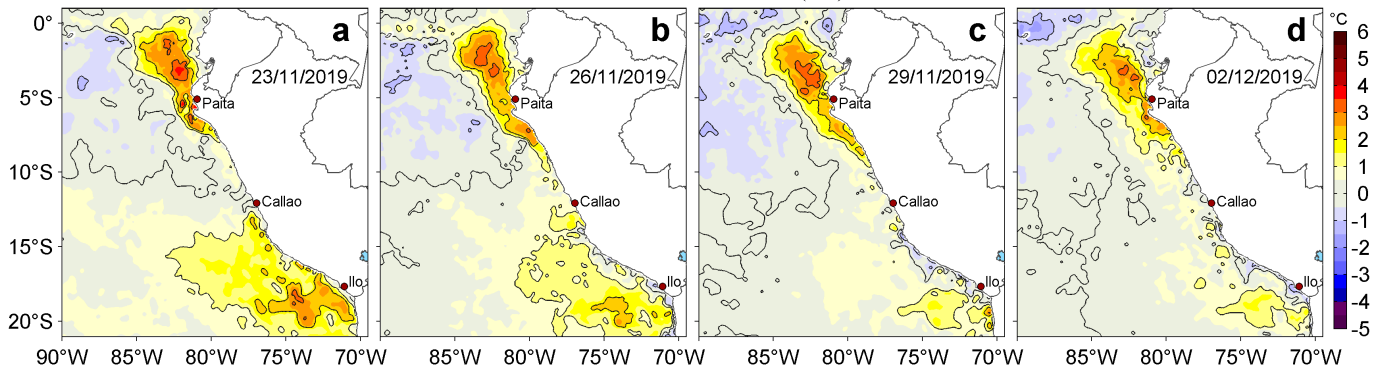
Figura 3. Anomalías de la temperatura superficial del mar (TSM, °C) para los días: a) 23, b) 26 y c) 29 de noviembre y d) 02 de diciembre de 2019. Las anomalías se calcularon respecto de la climatología para el periodo 2007-2016. Datos: OSTIA-UKMO-L4-GLOB-v2.0 (UK Met Office, 2012; Donlon et al, 2012). Procesamiento: LHF/AFIOF/DGIOCC/IMARPE.
