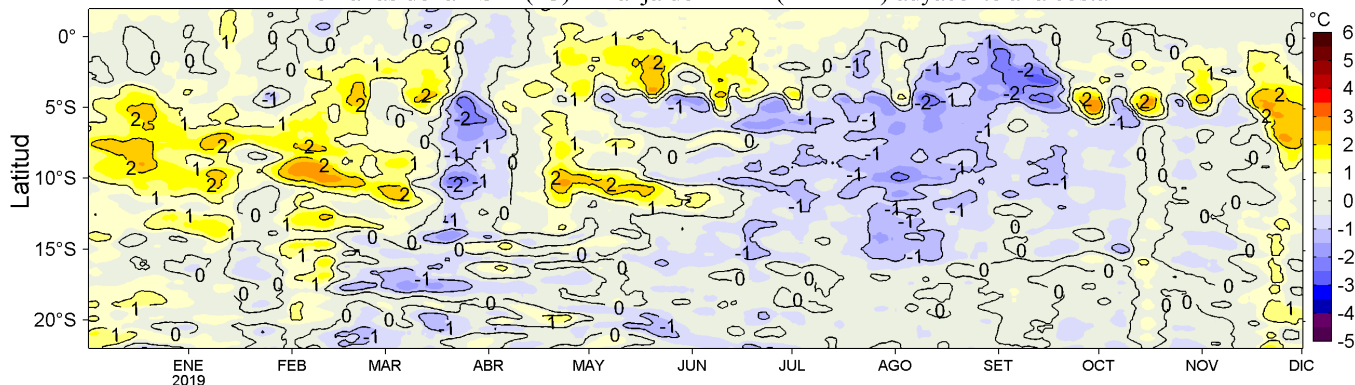
Figura 4. Variación promedio de las anomalías de la temperatura superficial del mar (TSM, °C) para una franja de 60 mn (~111 km) adyacente al litoral peruano para los últimos doce meses al 01 de diciembre de 2019. Datos: OSTIA-UKMO-L4-GLOB-v2.0 (UK Met. Office, 2012; Donlon et al, 2012) disponible en https://podaac.jpl.nasa.gov/dataset/OSTIA-UKMO-L4-GLOB-v2.0 . Las anomalías se calcularon con respecto al periodo 2007-2016. Procesamiento: LHF/AFIOF/DGIOCC/IMARPE.
