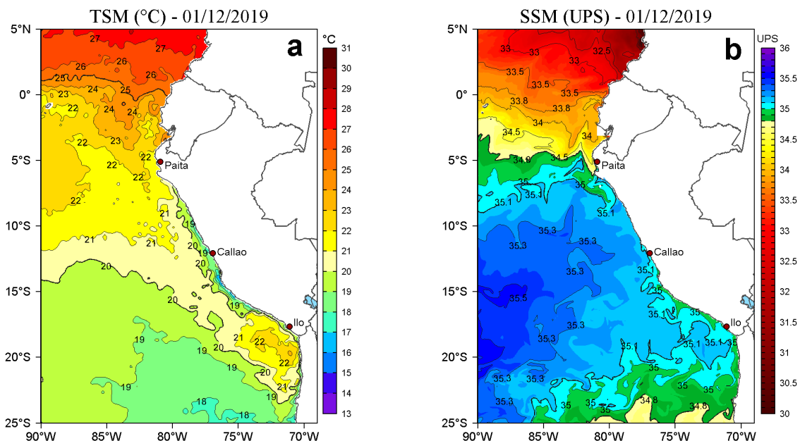
Figura 2. a) Temperatura superficial del mar (TSM, °C) y b) Salinidad superficial del mar (SSM, UPS), para el 01 de diciembre de 2019. Datos: OSTIA-UKMO-L4-GLOB-v2.0 (UK Met Office, 2012; Donlon et al, 2012) disponible en https://podaac.jpl.nasa.gov/dataset/OSTIA-UKMO-L4-GLOB-v2.0 para (a) y Hybrid Coordinate Ocean Model v. GOFS 3.1 (HYCOM; Halliwell et al., 1998; 2000; Bleck, 2001) para (b). Procesamiento: LHF/AFIOF/DGIOCC/IMARPE.
