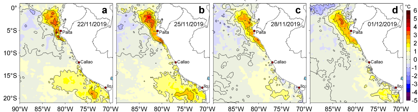
Figura 3. Anomalías de la temperatura superficial del mar (TSM, °C) para los días: a) 22, b) 25 y c) 28 de noviembre y d) 01 de diciembre de 2019. Las anomalías se calcularon respecto de la climatología para el periodo 2007-2016. Datos: OSTIA-UKMO-L4-GLOB-v2.0 (UK Met Office, 2012; Donlon et al, 2012). Procesamiento: LHF/AFIOF/DGIOCC/IMARPE.
