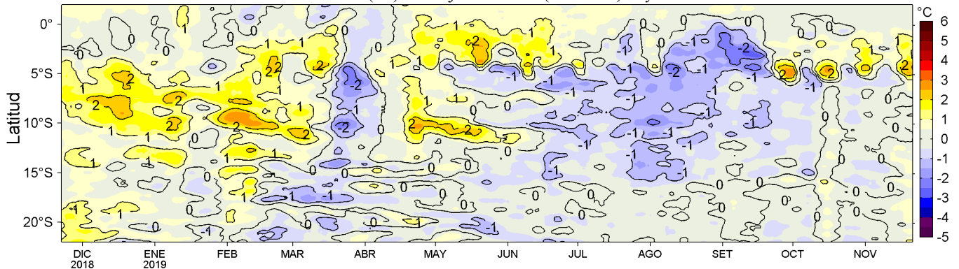
Figura 4. Variación promedio de las anomalías de la temperatura superficial del mar (TSM, °C) para una franja de 60 mn (~111 km) adyacente al litoral peruano para los últimos doce meses al 21 de noviembre de 2019. Datos: OSTIA-UKMO-L4-GLOB-v2.0 (UK Met. Office, 2012; Donlon et al, 2012) disponible en https://podaac.jpl.nasa.gov/dataset/OSTIA-UKMO-L4-GLOB-v2.0 . Las anomalías se calcularon con respecto al periodo 2007-2016. Procesamiento: LHF/AFIOF/DGIOCC/IMARPE.
