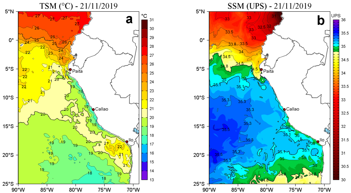
Figura 2. a) Temperatura superficial del mar (TSM, °C) y b) Salinidad superficial del mar (SSM, UPS), para el 21 de noviembre de 2019. Datos: OSTIA-UKMO-L4-GLOB-v2.0 (UK Met Office, 2012; Donlon et al, 2012) disponible en https://podaac.jpl.nasa.gov/dataset/OSTIA-UKMO-L4-GLOB-v2.0 para (a) y Hybrid Coordinate Ocean Model v. GOFS 3.1 (HYCOM; Halliwell et al., 1998; 2000; Bleck, 2001) para (b). Procesamiento: LHF/AFIOF/DGIOCC/IMARPE.
