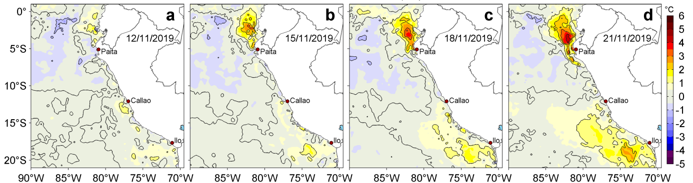
Figura 3. Anomalías de la temperatura superficial del mar (TSM, °C) para los días: a) 12, b) 15, c) 18 y d) 21 de noviembre de 2019. Las anomalías se calcularon respecto de la climatología para el periodo 2007-2016. Datos: OSTIA-UKMO-L4-GLOB-v2.0 (UK Met Office, 2012; Donlon et al, 2012). Procesamiento: LHF/AFIOF/DGIOCC/IMARPE.
