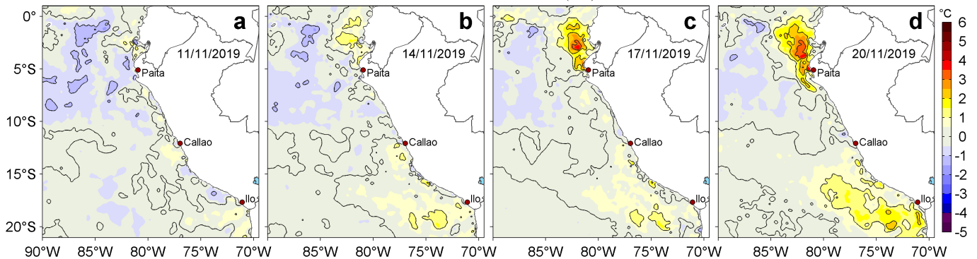
Figura 3. Anomalías de la temperatura superficial del mar (TSM, °C) para los días: a) 11, b) 14, c) 17 y d) 20 de noviembre de 2019. Las anomalías se calcularon respecto de la climatología para el periodo 2007-2016. Datos: OSTIA-UKMO-L4-GLOB-v2.0 (UK Met Office, 2012; Donlon et al, 2012). Procesamiento: LHF/AFIOF/DGIOCC/IMARPE.
