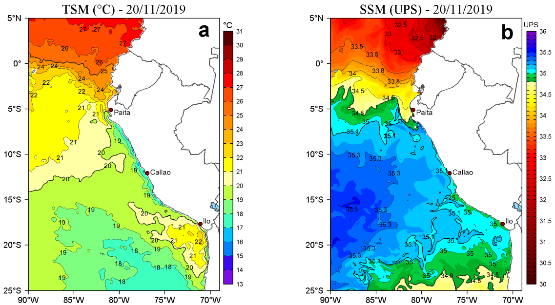
Figura 2. a) Temperatura superficial del mar (TSM, °C) y b) Salinidad superficial del mar (SSM, UPS), para el 20 de noviembre de 2019. Datos: OSTIA-UKMO-L4-GLOB-v2.0 (UK Met Office, 2012; Donlon et al, 2012) disponible en https://podaac.jpl.nasa.gov/dataset/OSTIA-UKMO-L4-GLOB-v2.0 para (a) y Hybrid Coordinate Ocean Model v. GOFS 3.1 (HYCOM; Halliwell et al., 1998; 2000; Bleck, 2001) para (b). Procesamiento: LHF/AFIOF/DGIOCC/IMARPE.
