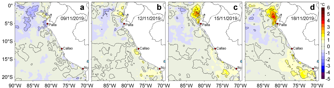
Figura 3. Anomalías de la temperatura superficial del mar (TSM, °C) para los días: a) 09, b) 12, c) 15 y d) 18 de noviembre de 2019. Las anomalías se calcularon respecto de la climatología para el periodo 2007-2016. Datos: OSTIA-UKMO-L4-GLOB-v2.0 (UK Met Office, 2012; Donlon et al, 2012). Procesamiento: LHF/AFIOF/DGIOCC/IMARPE.
