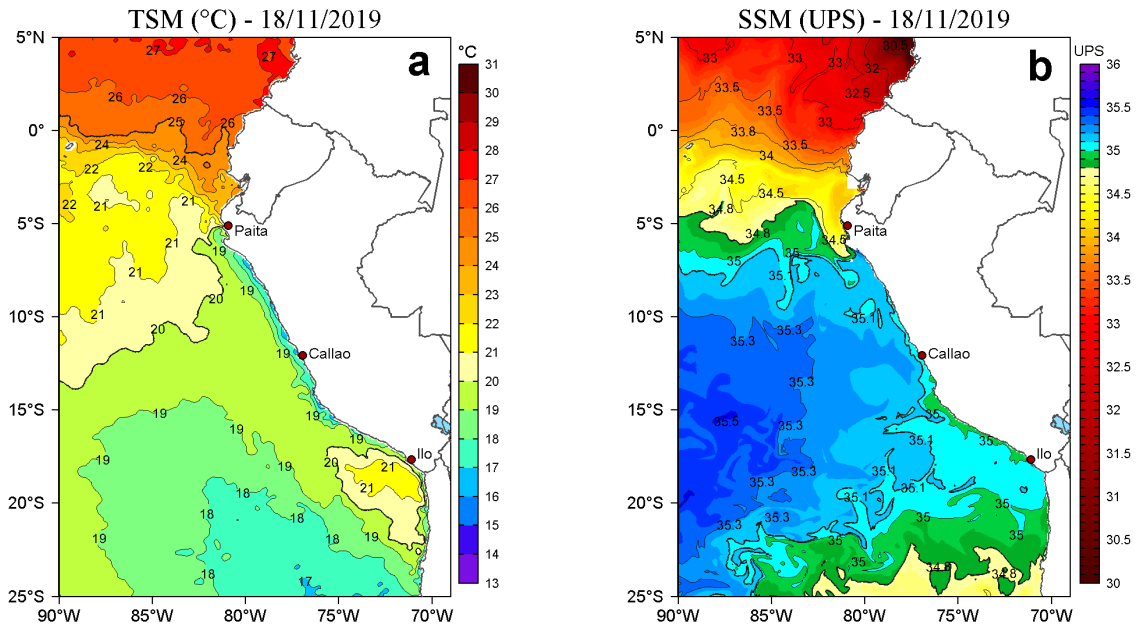
Figura 2. a) Temperatura superficial del mar (TSM, °C) y b) Salinidad superficial del mar (SSM, UPS), para el 18 de noviembre de 2019. Datos: OSTIA-UKMO-L4-GLOB-v2.0 (UK Met Office, 2012; Donlon et al, 2012) disponible en https://podaac.jpl.nasa.gov/dataset/OSTIA-UKMO-L4-GLOB-v2.0 para (a) y Hybrid Coordinate Ocean Model v. GOFS 3.1 (HYCOM; Halliwell et al., 1998; 2000; Bleck, 2001) para (b). Procesamiento: LHF/AFIOF/DGIOCC/IMARPE.
