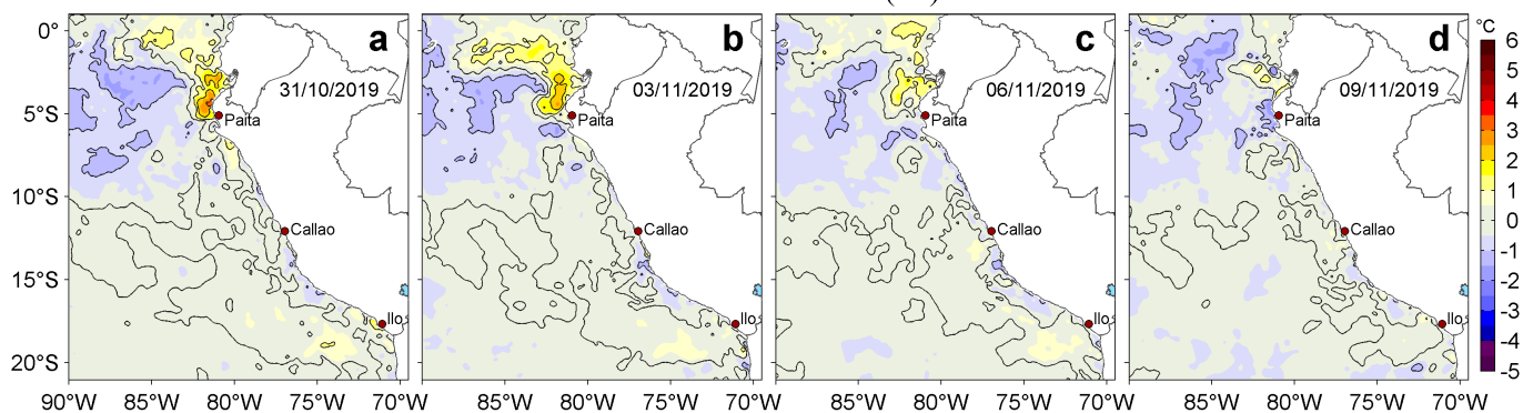
Figura 3. Anomalías de la temperatura superficial del mar (TSM, °C) para los días: a) 31 de octubre, b) 03, c) 06 y d) 09 de noviembre de 2019. Las anomalías se calcularon respecto de la climatología para el periodo 2007-2016. Datos: OSTIA-UKMO-L4-GLOB-v2.0 (UK Met Office, 2012; Donlon et al, 2012). Procesamiento: LHF/AFIOF/DGIOCC/IMARPE.
