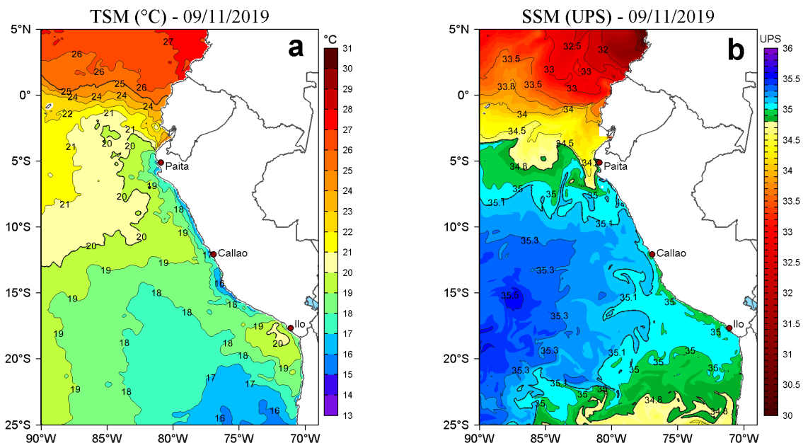
Figura 2. a) Temperatura superficial del mar (TSM, °C) y b) Salinidad superficial del mar (SSM, UPS), para el 09 de noviembre de 2019. Datos: OSTIA-UKMO-L4-GLOB-v2.0 (UK Met Office, 2012; Donlon et al, 2012) disponible en https://podaac.jpl.nasa.gov/dataset/OSTIA-UKMO-L4-GLOB-v2.0 para (a) y Hybrid Coordinate Ocean Model v. GOF3.1 (HYCOM; Halliwell et al., 1998; 2000; Bleck, 2001) para (b). Procesamiento: LHF/AFIOF/DGIOCC/IMARPE.
