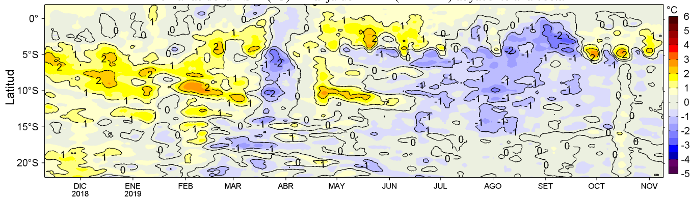
Figura 4. Variación promedio de las anomalías de la temperatura superficial del mar (TSM, °C) para una franja de 60 mn (~111 km) adyacente al litoral peruano para los últimos doce meses al 09 de noviembre de 2019. Datos: OSTIA-UKMO-L4-GLOB-v2.0 (UK Met. Office, 2012; Donlon et al, 2012) disponible en https://podaac.jpl.nasa.gov/dataset/OSTIA-UKMO-L4-GLOB-v2.0 . Las anomalías se calcularon con respecto al periodo 2007-2016. Procesamiento: LHF/AFIOF/DGIOCC/IMARPE.
