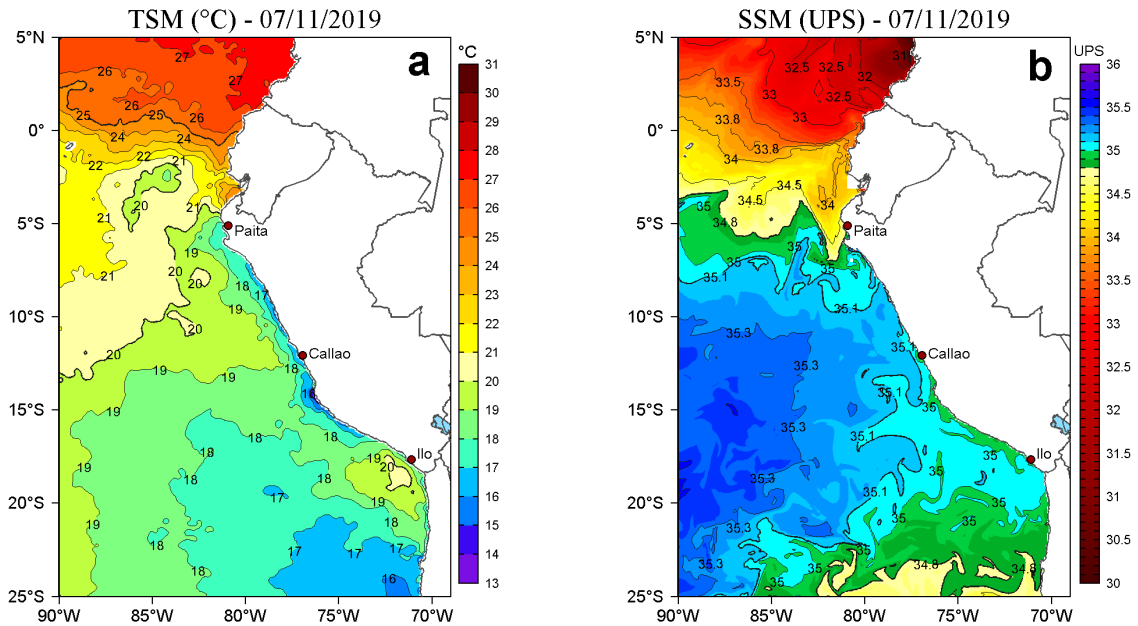
Figura 2. a) Temperatura superficial del mar (TSM, °C) y b) Salinidad superficial del mar (SSM, UPS), para el 07 de noviembre de 2019. Datos: OSTIA-UKMO-L4-GLOB-v2.0 (UK Met Office, 2012; Donlon et al, 2012) disponible en https://podaac.jpl.nasa.gov/dataset/OSTIA-UKMO-L4-GLOB-v2.0 para (a) y Hybrid Coordinate Ocean Model v. GOFS 3.1 (HYCOM; Halliwell et al., 1998; 2000; Bleck, 2001) para (b). Procesamiento: LHF/AFIOF/DGIOCC/IMARPE.
