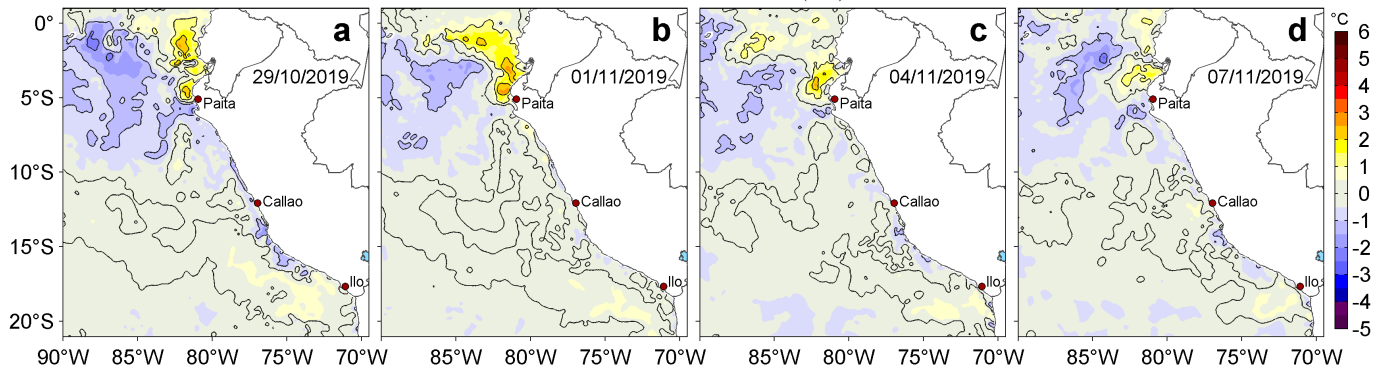
Figura 3. Anomalías de la temperatura superficial del mar (TSM, °C) para los días: a) 29 de octubre, b) 01, c) 04 y d) 07 de noviembre de 2019. Las anomalías se calcularon respecto de la climatología para el periodo 2007-2016. Datos: OSTIA-UKMO-L4-GLOB-v2.0 (UK Met Office, 2012; Donlon et al, 2012). Procesamiento: LHF/AFIOF/DGIOCC/IMARPE.
