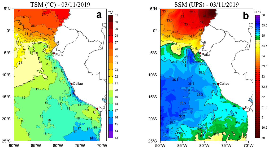
Figura 2. a) Temperatura superficial del mar (TSM, °C) y b) Salinidad superficial del mar (SSM, UPS), para el 03 de noviembre de 2019. Datos: OSTIA-UKMO-L4-GLOB-v2.0 (UK Met Office, 2012; Donlon et al, 2012) disponible en https://podaac.jpl.nasa.gov/dataset/OSTIA-UKMO-L4-GLOB-v2.0 para (a) y Hybrid Coordinate Ocean Model v. GOFS 3.1 (HYCOM; Halliwell et al., 1998; 2000; Bleck, 2001) para (b). Procesamiento: LHF/AFIOF/DGIOCC/IMARPE.
