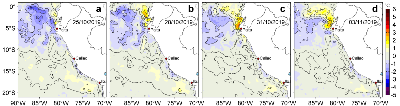
Figura 3. Anomalías de la temperatura superficial del mar (TSM, °C) para los días: a) 25, b) 28 y c) 31 de octubre y d) 03 de noviembre de 2019. Las anomalías se calcularon respecto de la climatología para el periodo 2007-2016. Datos: OSTIA-UKMO-L4-GLOB-v2.0 (UK Met Office, 2012; Donlon et al, 2012). Procesamiento: LHF/AFIOF/DGIOCC/IMARPE.
