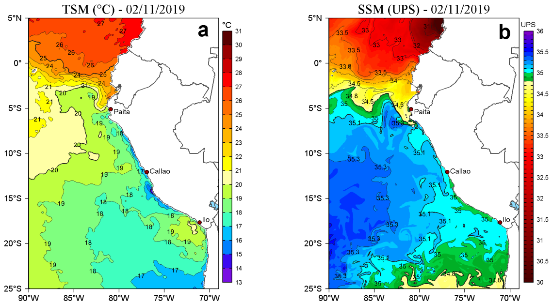
Figura 2. a) Temperatura superficial del mar (TSM, °C) y b) Salinidad superficial del mar (SSM, UPS), para el 02 de noviembre de 2019. Datos: OSTIA-UKMO-L4-GLOB-v2.0 (UK Met Office, 2012; Donlon et al, 2012) disponible en https://podaac.jpl.nasa.gov/dataset/OSTIA-UKMO-L4-GLOB-v2.0 para (a) y Hybrid Coordinate Ocean Model v. GOFS 3.1 (HYCOM; Halliwell et al., 1998; 2000; Bleck, 2001) para (b). Procesamiento: LHF/AFIOF/DGIOCC/IMARPE.
