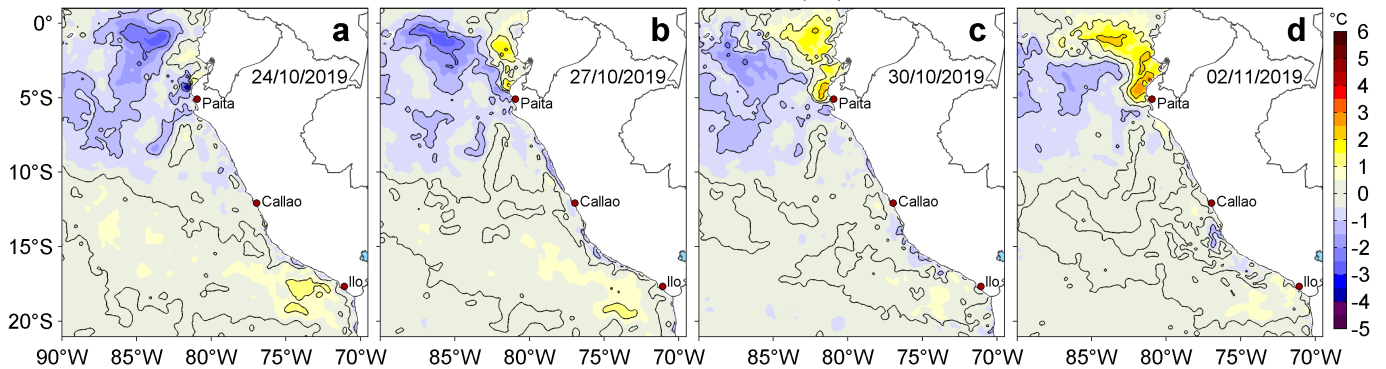
Figura 3. Anomalías de la temperatura superficial del mar (TSM, °C) para los días: a) 24, b) 27 y c) 30 de octubre y d) 02 de noviembre de 2019. Las anomalías se calcularon respecto de la climatología para el periodo 2007-2016. Datos: OSTIA-UKMO-L4-GLOB-v2.0 (UK Met Office, 2012; Donlon et al, 2012). Procesamiento: LHF/AFIOF/DGIOCC/IMARPE.
