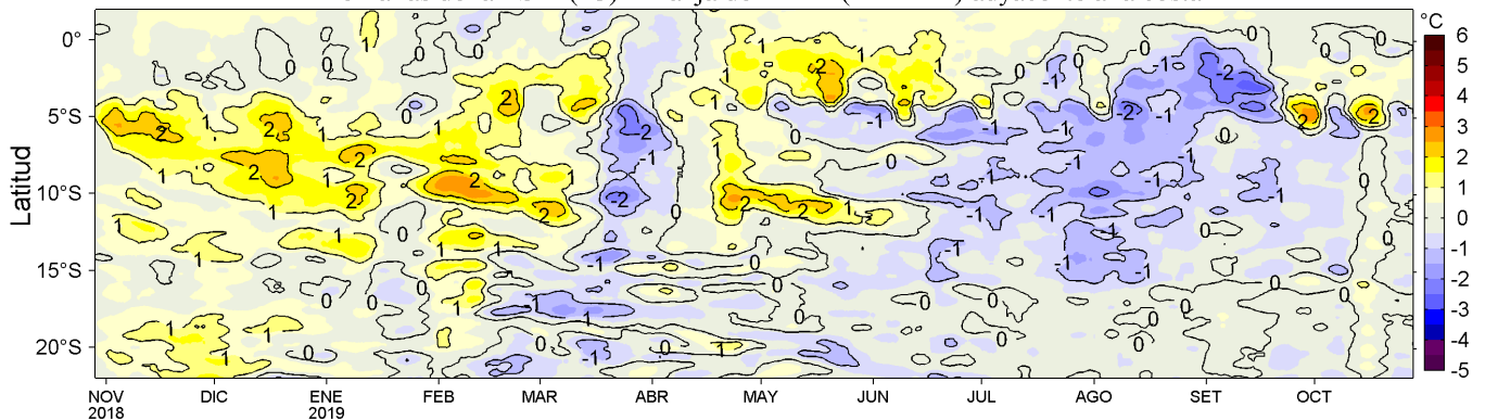
Figura 4. Variación promedio de las anomalías de la temperatura superficial del mar (TSM, °C) para una franja de 60 mn (~111 km) adyacente al litoral peruano para los últimos doce meses al 28 de octubre de 2019. Datos: OSTIA-UKMO-L4-GLOB-v2.0 (UK Met. Office, 2012; Donlon et al, 2012) disponible en https://podaac.jpl.nasa.gov/dataset/OSTIA-UKMO-L4-GLOB-v2.0 . Las anomalías se calcularon con respecto al periodo 2007-2016. Procesamiento: LHF/AFIOF/DGIOCC/IMARPE.
