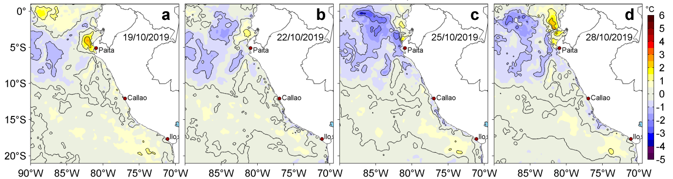
Figura 3. Anomalías de la temperatura superficial del mar (TSM, °C) para los días: a) 19, b) 22, c) 25 y d) 28 de octubre de 2019. Las anomalías se calcularon respecto de la climatología para el periodo 2007-2016. Datos: OSTIA-UKMO-L4-GLOB-v2.0 (UK Met Office, 2012; Donlon et al, 2012). Procesamiento: LHF/AFIOF/DGIOCC/IMARPE.
