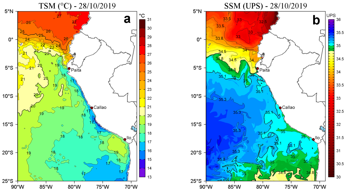
Figura 2. a) Temperatura superficial del mar (TSM, °C) y b) Salinidad superficial del mar (SSM, UPS), para el 28 de octubre de 2019. Datos: OSTIA-UKMO-L4-GLOB-v2.0 (UK Met Office, 2012; Donlon et al, 2012) disponible en https://podaac.jpl.nasa.gov/dataset/OSTIA-UKMO-L4-GLOB-v2.0 para (a) y Hybrid Coordinate Ocean Model v. GOF3 3.1 (HYCOM; Halliwell et al., 1998; 2000; Bleck, 2001) para (b). Procesamiento: LHF/AFIOF/DGIOCC/IMARPE.
