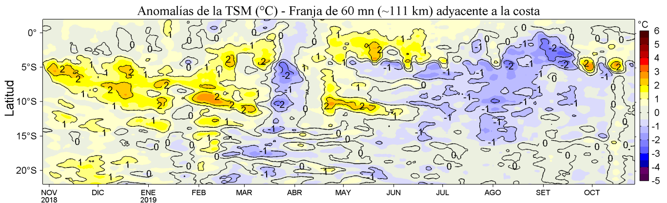
Figura 4. Variación promedio de las anomalías de la temperatura superficial del mar (TSM, °C) para una franja de 60 mn (~111 km) adyacente al litoral peruano para los últimos doce meses al 27 de octubre de 2019. Datos: OSTIA-UKMO-L4-GLOB-v2.0 (UK Met. Office, 2012; Donlon et al, 2012) disponible en https://podaac.jpl.nasa.gov/dataset/OSTIA-UKMO-L4-GLOB-v2.0 . Las anomalías se calcularon con respecto al periodo 2007-2016. Procesamiento: LHF/AFIOF/DGIOCC/IMARPE.
