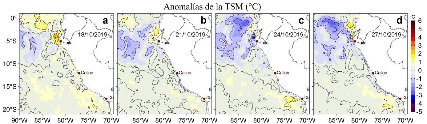
Figura 3. Anomalías de la temperatura superficial del mar (TSM, °C) para los días: a) 18, b) 21, c) 24 y d) 27 de octubre de 2019. Las anomalías se calcularon respecto de la climatología para el periodo 2007-2016. Datos: OSTIA-UKMO-L4-GLOB-v2.0 (UK Met Office, 2012; Donlon et al, 2012). Procesamiento: LHF/AFIOF/DGIOCC/IMARPE.
