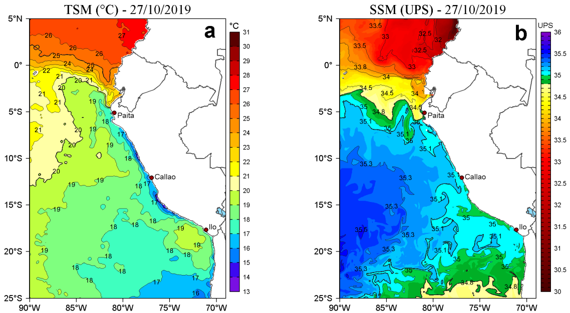
Figura 2. a) Temperatura superficial del mar (TSM, °C) y b) Salinidad superficial del mar (SSM, UPS), para el 27 de octubre de 2019. Datos: OSTIA-UKMO-L4-GLOB-v2.0 (UK Met Office, 2012; Donlon et al, 2012) disponible en https://podaac.jpl.nasa.gov/dataset/OSTIA-UKMO-L4-GLOB-v2.0 para (a) y Hybrid Coordinate Ocean Model v. GOF3 3.1 (HYCOM; Halliwell et al., 1998; 2000; Bleck, 2001) para (b). Procesamiento: LHF/AFIOF/DGIOCC/IMARPE.
