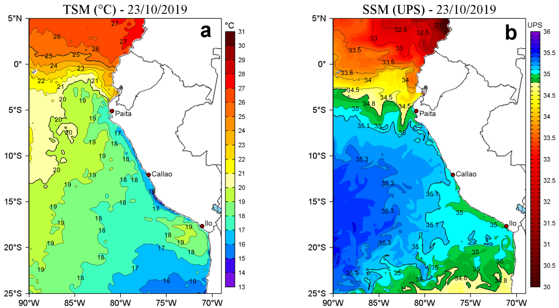
Figura 2. a) Temperatura superficial del mar (TSM, °C) y b) Salinidad superficial del mar (SSM, UPS), para el 23 de octubre de 2019. Datos: OSTIA-UKMO-L4-GLOB-v2.0 (UK Met Office, 2012; Donlon et al, 2012) disponible en https://podaac.jpl.nasa.gov/dataset/OSTIA-UKMO-L4-GLOB-v2.0 para (a) y Hybrid Coordinate Ocean Model v. GOF3 3.1 (HYCOM; Halliwell et al., 1998; 2000; Bleck, 2001) para (b). Procesamiento: LHF/AFIOF/DGIOCC/IMARPE.
