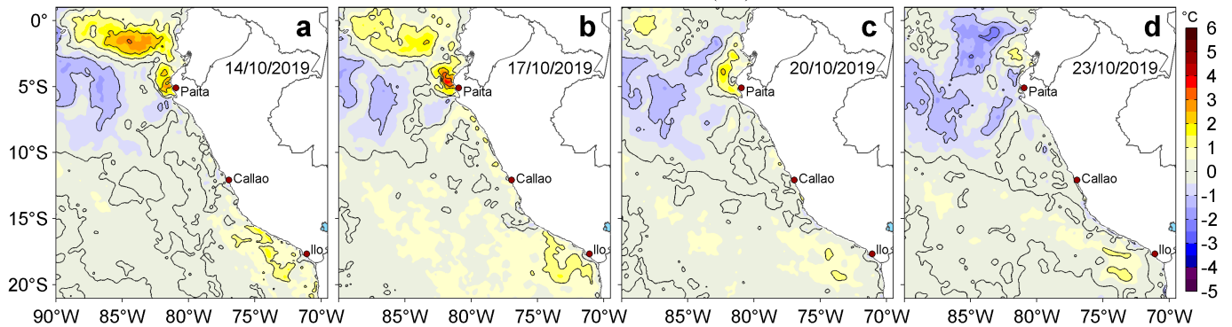
Figura 3. Anomalías de la temperatura superficial del mar (TSM, °C) para los días: a) 14, b) 17, c) 20 y d) 23 de octubre de 2019. Las anomalías se calcularon respecto de la climatología para el periodo 2007-2016. Datos: OSTIA-UKMO-L4-GLOB-v2.0 (UK Met Office, 2012; Donlon et al, 2012). Procesamiento: LHF/AFIOF/DGIOCC/IMARPE.
