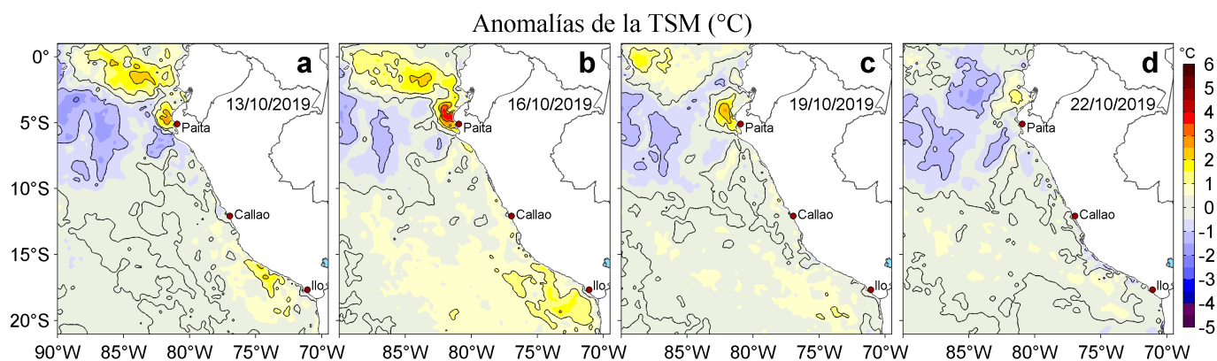
Figura 3. Anomalías de la temperatura superficial del mar (TSM, °C) para los días: a) 13, b) 16, c) 19 y d) 22 de octubre de 2019. Las anomalías se calcularon respecto de la climatología para el periodo 2007-2016. Datos: OSTIA-UKMO-L4-GLOB-v2.0 (UK Met Office, 2012; Donlon et al, 2012). Procesamiento: LHF/AFIOF/DGIOCC/IMARPE.
