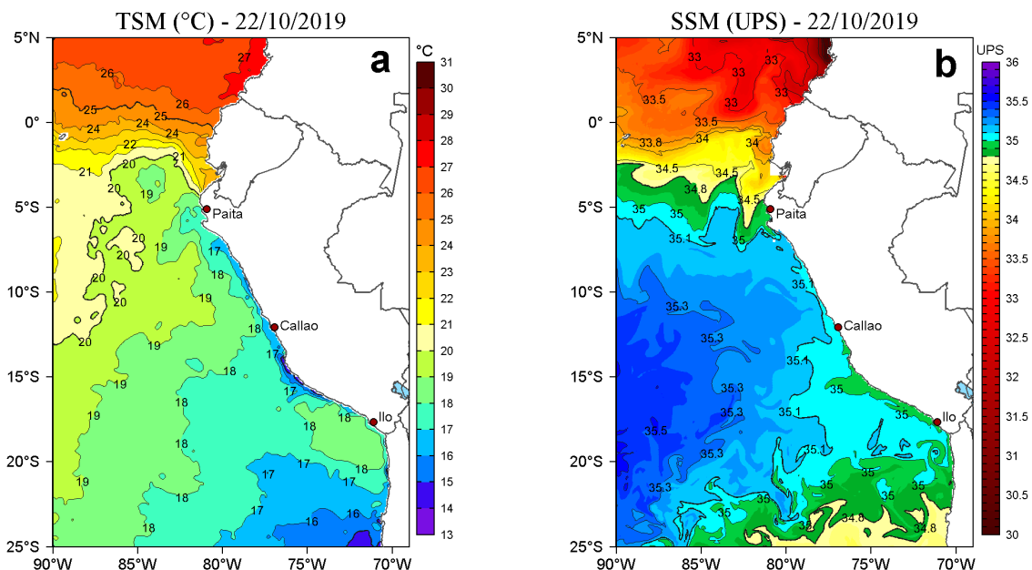
Figura 2. a) Temperatura superficial del mar (TSM, °C) y b) Salinidad superficial del mar (SSM, UPS), para el 22 de octubre de 2019. Datos: OSTIA-UKMO-L4-GLOB-v2.0 (UK Met Office, 2012; Donlon et al, 2012) disponible en https://podaac.jpl.nasa.gov/dataset/OSTIA-UKMO-L4-GLOB-v2.0 para (a) y Hybrid Coordinate Ocean Model v. GOF3 3.1 (HYCOM; Halliwell et al., 1998; 2000; Bleck, 2001) para (b). Procesamiento: LHF/AFIOF/DGIOCC/IMARPE.
