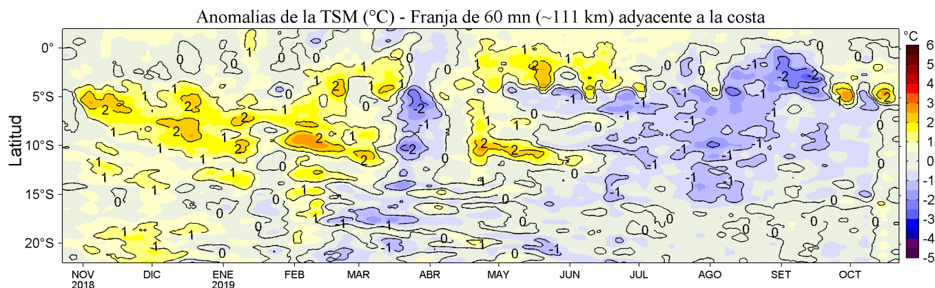
Figura 4. Variación promedio de las anomalías de la temperatura superficial del mar (TSM, °C) para una franja de 60 mn (~111 km) adyacente al litoral peruano para los últimos doce meses al 22 de octubre de 2019. Datos: OSTIA-UKMO-L4-GLOB-v2.0 (UK Met. Office, 2012; Donlon et al, 2012) disponible en https://podaac.jpl.nasa.gov/dataset/OSTIA-UKMO-L4-GLOB-v2.0 . Las anomalías se calcularon con respecto al periodo 2007-2016. Procesamiento: LHF/AFIOF/DGIOCC/IMARPE.
