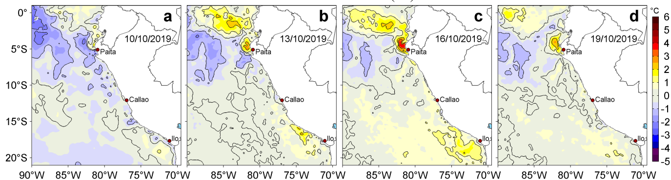
Figura 3. Anomalías de la temperatura superficial del mar (TSM, °C) para los días: a) 10, b) 13, c) 16 y d) 19 de octubre de 2019. Las anomalías se calcularon respecto de la climatología para el periodo 2007-2016. Datos: OSTIA-UKMO-L4-GLOB-v2.0 (UK Met Office, 2012; Donlon et al, 2012). Procesamiento: LHF/AFIOF/DGIOCC/IMARPE.
