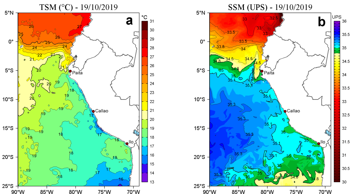
Figura 2. a) Temperatura superficial del mar (TSM, °C) y b) Salinidad superficial del mar (SSM, UPS), para el 19 de octubre de 2019. Datos: OSTIA-UKMO-L4-GLOB-v2.0 (UK Met Office, 2012; Donlon et al, 2012) disponible en https://podaac.jpl.nasa.gov/dataset/OSTIA-UKMO-L4-GLOB-v2.0 para (a) y Hybrid Coordinate Ocean Model v. GOF3 3.1 (HYCOM; Halliwell et al., 1998; 2000; Bleck, 2001) para (b). Procesamiento: LHF/AFIOF/DGIOCC/IMARPE.
