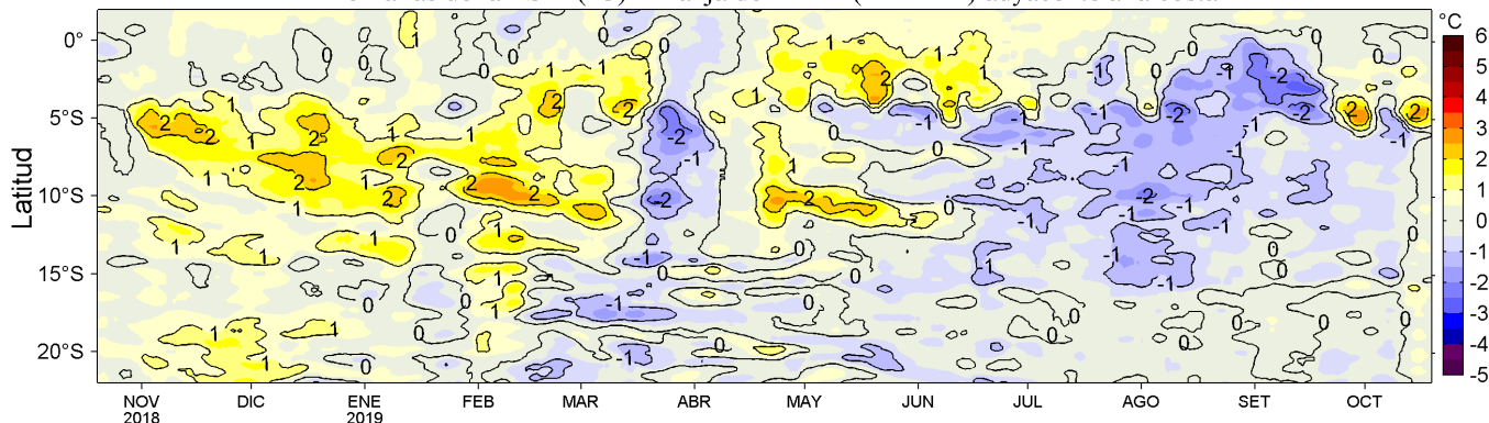
Figura 4. Variación promedio de las anomalías de la temperatura superficial del mar (TSM, °C) para una franja de 60 mn (~111 km) adyacente al litoral peruano para los últimos doce meses al 19 de octubre de 2019. Datos: OSTIA-UKMO-L4-GLOB-v2.0 (UK Met. Office, 2012; Donlon et al, 2012) disponible en https://podaac.jpl.nasa.gov/dataset/OSTIA-UKMO-L4-GLOB-v2.0 . Las anomalías se calcularon con respecto al periodo 2007-2016. Procesamiento: LHF/AFIOF/DGIOCC/IMARPE.
