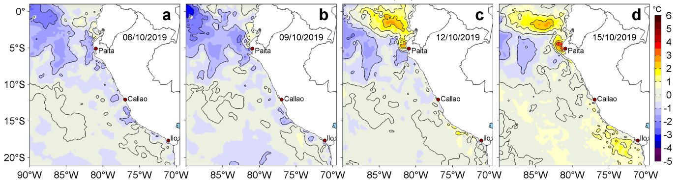
Figura 3. Anomalías de la temperatura superficial del mar (TSM, °C) para los días: a) 06, b) 09, c) 12 y d) 15 de octubre de 2019. Las anomalías se calcularon respecto de la climatología para el periodo 2007-2016. Datos: OSTIA-UKMO-L4-GLOB-v2.0 (UK Met Office, 2012; Donlon et al, 2012). Procesamiento: LHF/AFIOF/DGIOCC/IMARPE.
