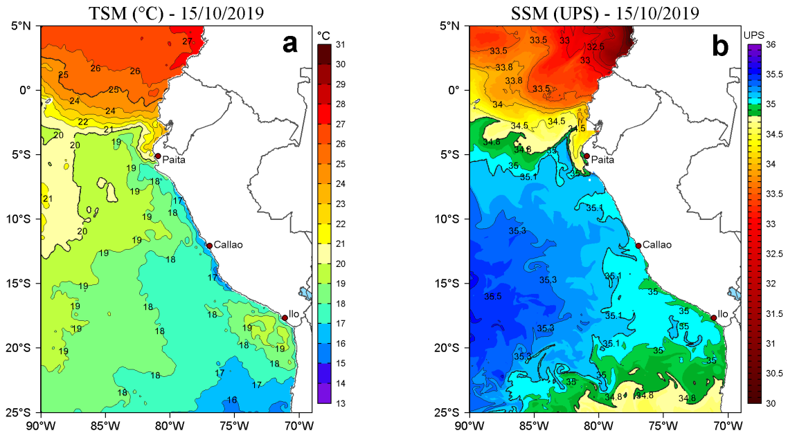
Figura 2. a) Temperatura superficial del mar (TSM, °C) y b) Salinidad superficial del mar (SSM, UPS), para el 15 de octubre de 2019. Datos: OSTIA-UKMO-L4-GLOB-v2.0 (UK Met Office, 2012; Donlon et al, 2012) disponible en https://podaac.jpl.nasa.gov/dataset/OSTIA-UKMO-L4-GLOB-v2.0 para (a) y Hybrid Coordinate Ocean Model v. GOF3 3.1 (HYCOM; Halliwell et al., 1998; 2000; Bleck, 2001) para (b). Procesamiento: LHF/AFIOF/DGIOCC/IMARPE.
