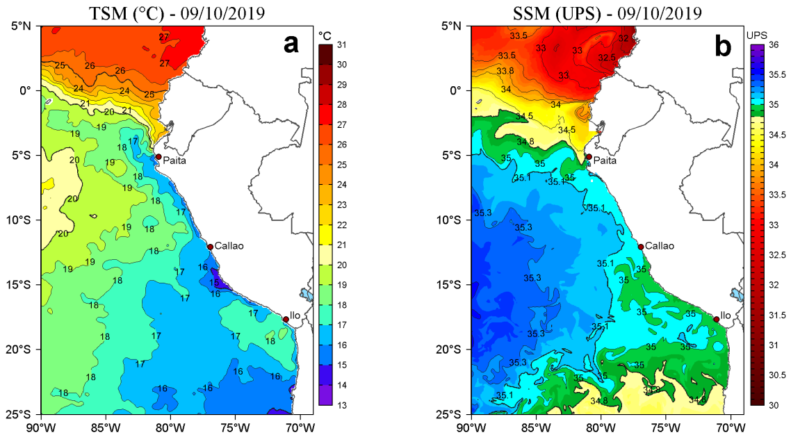
Figura 2. a) Temperatura superficial del mar (TSM, °C) y b) Salinidad superficial del mar (SSM, UPS), para el 09 de octubre de 2019. Datos: OSTIA-UKMO-L4-GLOB-v2.0 (UK Met Office, 2012; Donlon et al, 2012) disponible en https://podaac.jpl.nasa.gov/dataset/OSTIA-UKMO-L4-GLOB-v2.0 para (a) y Hybrid Coordinate Ocean Model v. GOF3 3.1 (HYCOM; Halliwell et al., 1998; 2000; Bleck, 2001) para (b). Procesamiento: LHF/AFIOF/DGIOCC/IMARPE.
