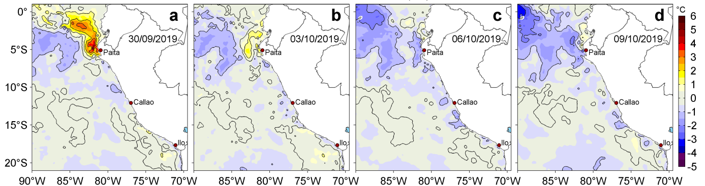
Figura 3. Anomalías de la temperatura superficial del mar (TSM, °C) para los días: a) 30 de setiembre, b) 03, c) 06 y d) 09 de octubre de 2019. Las anomalías se calcularon respecto de la climatología para el periodo 2007-2016. Datos: OSTIA-UKMO-L4-GLOB-v2.0 (UK Met Office, 2012; Donlon et al, 2012). Procesamiento: LHF/AFIOF/DGIOCC/IMARPE.
