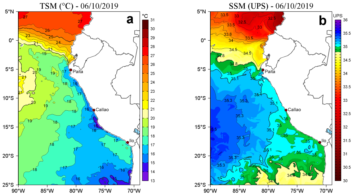
Figura 2. a) Temperatura superficial del mar (TSM, °C) y b) Salinidad superficial del mar (SSM, UPS), para el 06 de octubre de 2019. Datos: OSTIA-UKMO-L4-GLOB-v2.0 (UK Met Office, 2012; Donlon et al, 2012) disponible en https://podaac.jpl.nasa.gov/dataset/OSTIA-UKMO-L4-GLOB-v2.0 para (a) y Hybrid Coordinate Ocean Model v. GOF3 3.1 (HYCOM; Halliwell et al., 1998; 2000; Bleck, 2001) para (b). Procesamiento: LHF/AFIOF/DGIOCC/IMARPE.
