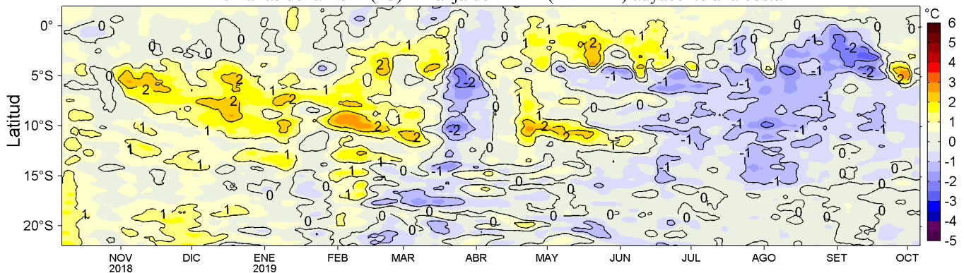
Figura 4. Variación promedio de las anomalías de la temperatura superficial del mar (TSM, °C) para una franja de 60 mn (~111 km) adyacente al litoral peruano para los últimos doce meses al 06 de octubre de 2019. Datos: OSTIA-UKMO-L4-GLOB-v2.0 (UK Met. Office, 2012; Donlon et al, 2012) disponible en https://podaac.jpl.nasa.gov/dataset/OSTIA-UKMO-L4-GLOB-v2.0 . Las anomalías se calcularon con respecto al periodo 2007-2016. Procesamiento: LHF/AFIOF/DGIOCC/IMARPE.
