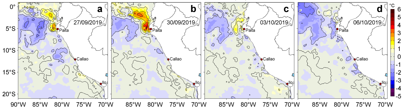
Figura 3. Anomalías de la temperatura superficial del mar (TSM, °C) para los días: a) 27 y b) 30 de setiembre, c) 03 y d) 06 de octubre de 2019. Las anomalías se calcularon respecto de la climatología para el periodo 2007-2016. Datos: OSTIA-UKMO-L4-GLOB-v2.0 (UK Met Office, 2012; Donlon et al, 2012). Procesamiento: LHF/AFIOF/DGIOCC/IMARPE.
