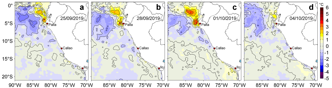
Figura 3. Anomalías de la temperatura superficial del mar (TSM, °C) para los días: a) 25 y b) 28 de setiembre, c) 01 y d) 04 de octubre de 2019. Las anomalías se calcularon respecto de la climatología para el periodo 2007-2016. Datos: OSTIA-UKMO-L4-GLOB-v2.0 (UK Met Office, 2012; Donlon et al, 2012). Procesamiento: LHF/AFIOF/DGIOCC/IMARPE.
