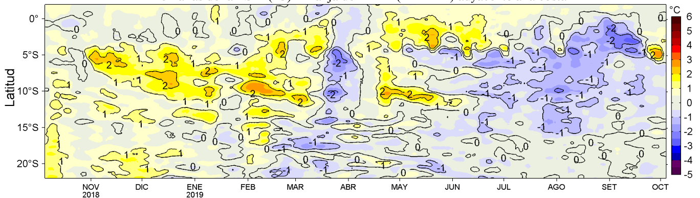
Figura 4. Variación promedio de las anomalías de la temperatura superficial del mar (TSM, °C) para una franja de 60 mn (~111 km) adyacente al litoral peruano para los últimos doce meses al 04 de octubre de 2019. Datos: OSTIA-UKMO-L4-GLOB-v2.0 (UK Met. Office, 2012; Donlon et al, 2012) disponible en https://podaac.jpl.nasa.gov/dataset/OSTIA-UKMO-L4-GLOB-v2.0 . Las anomalías se calcularon con respecto al periodo 2007-2016. Procesamiento: LHF/AFIOF/DGIOCC/IMARPE.
