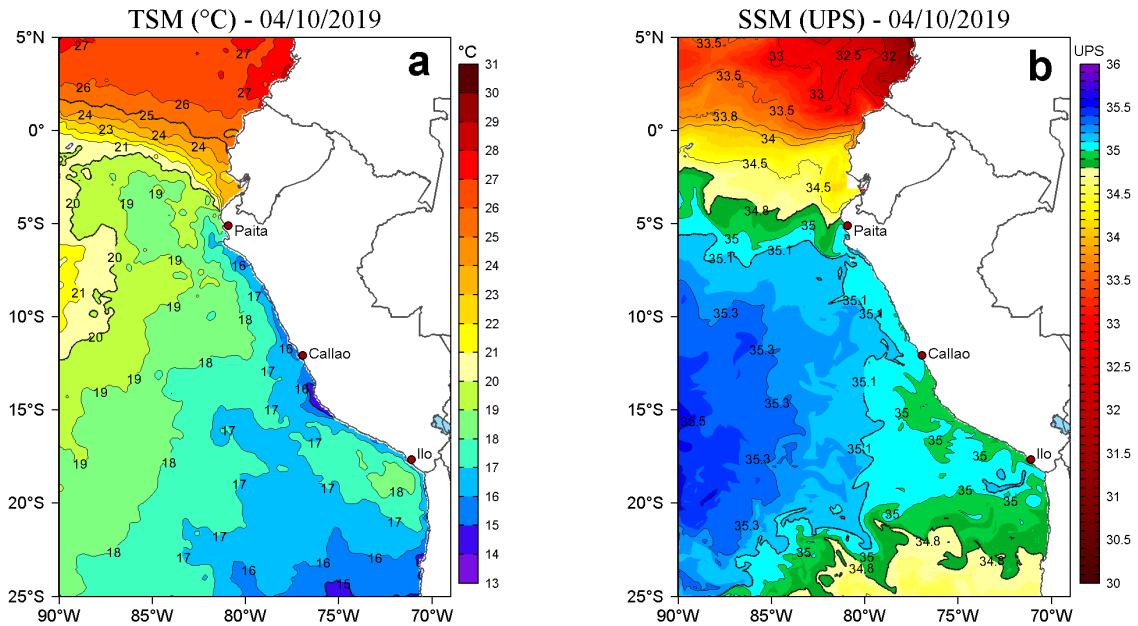
Figura 2. a) Temperatura superficial del mar (TSM, °C) y b) Salinidad superficial del mar (SSM, UPS), para el 04 de octubre de 2019. Datos: OSTIA-UKMO-L4-GLOB-v2.0 (UK Met Office, 2012; Donlon et al, 2012) disponible en https://podaac.jpl.nasa.gov/dataset/OSTIA-UKMO-L4-GLOB-v2.0 para (a) y Hybrid Coordinate Ocean Model v. GOF3 3.1 (HYCOM; Halliwell et al., 1998; 2000; Bleck, 2001) para (b). Procesamiento: LHF/AFIOF/DGIOCC/IMARPE.
